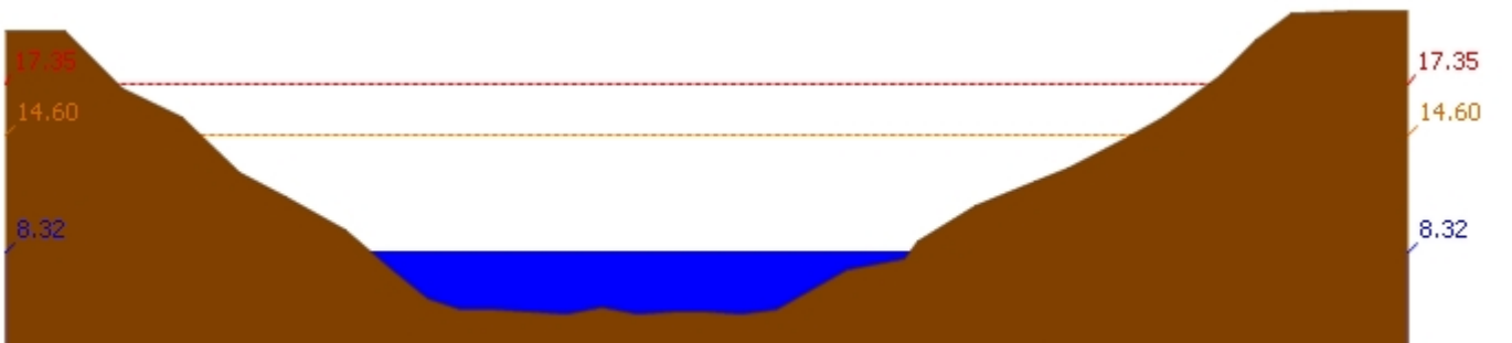
สถานี 120109T แม่น้ำป่าสักที่ อ.แก่งคอย ต.แก่งคอย อ.แก่งคอย จ.สระบุรี ระดับน้ำ 8.32 ม.รทก.
