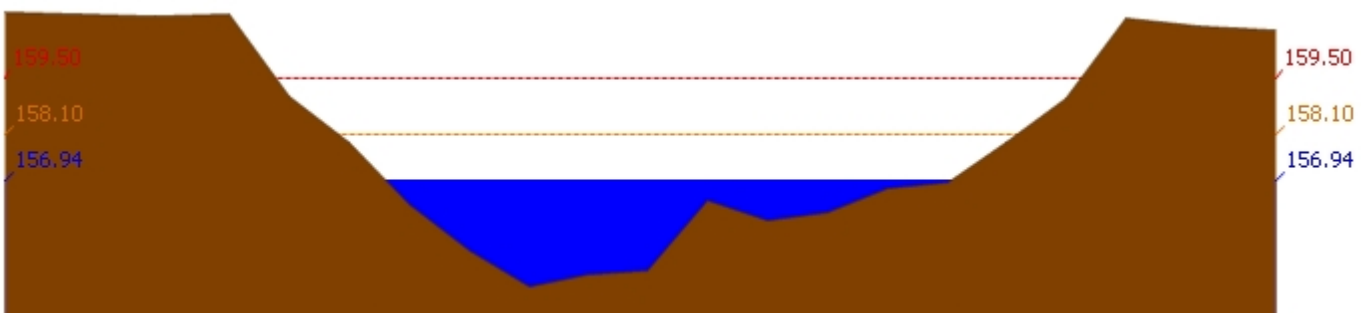
สถานี 120305T หัวน้ำพุที่ อ.หล่มเก่า ต.หล่มเก่า อ.หล่มเก่า จ.เพชรบูรณ์ ระดับน้ำ 156.94 ม.รทก.
