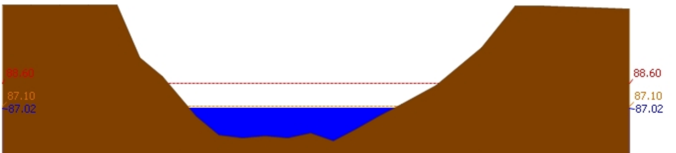
สถานี 120110T แม่น้ำป่าสักที่บ้านวังโบสถ์ ต.วังโบสถ์ อ.หนองไผ่ จ.เพชรบูรณ์ ระดับน้ำ 87.02 ม.รทก.
