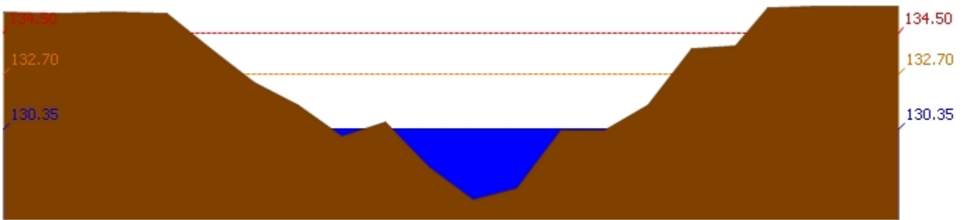
สถานี 120111T แม่น้ำป่าสักที่บ้านจางวาง ต.ลานบัว อ.หล่มสัก จ.เพชรบูรณ์ ระดับน้ำ 130.35 ม.รทก.
