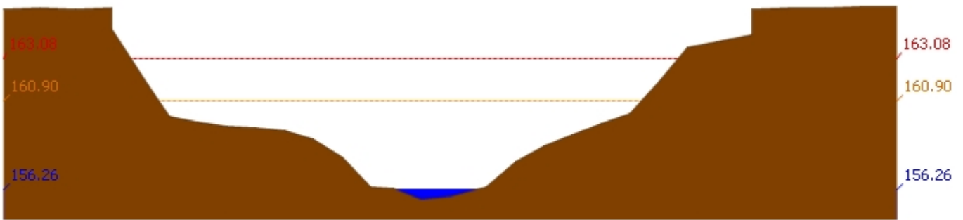
สถานี 120105T แม่น้ำป่าสักที่บ้านวังมเสหนือ ต.ท่าอิบุญ อ.หล่มสัก จ.เพชรบูรณ์ ระดับน้ำ 156.26 ม.รทก.
