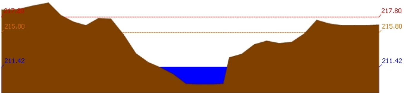
สถานี 120205T แม่น้ำป่าสักที่บ้านอู่กะทาด ต.ศิลา อ.หล่มเก่า จ.เพชรบูรณ์ ระดับน้ำ 211.42 ม.รทก.
