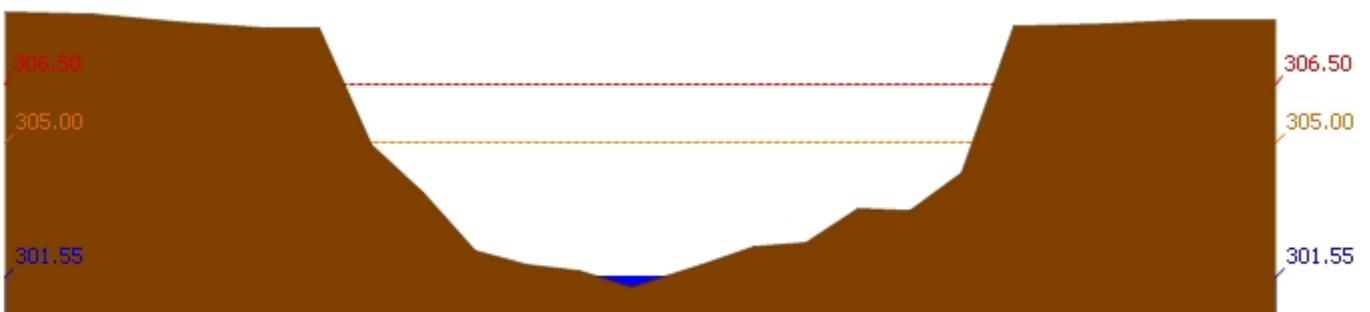
สถานี 120304T หัวน้ำพุที่บ้านกกกะบาก ต.โป่ง อ.ด่านซ้าย จ.เลย ระดับน้ำ 301.55 ม.รทก.
