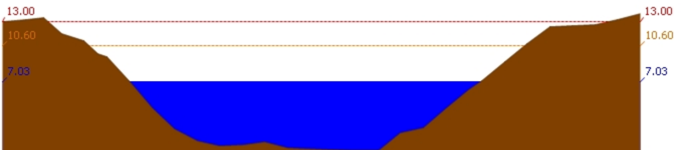
สถานี 120106T แม่น้ำป่าสักที่ อ.เสนาห์ ต.ศาลาวิไทย อ.เสนาห์ จ.สระบุรี ระดับน้ำ 7.03 ม.รทก.
