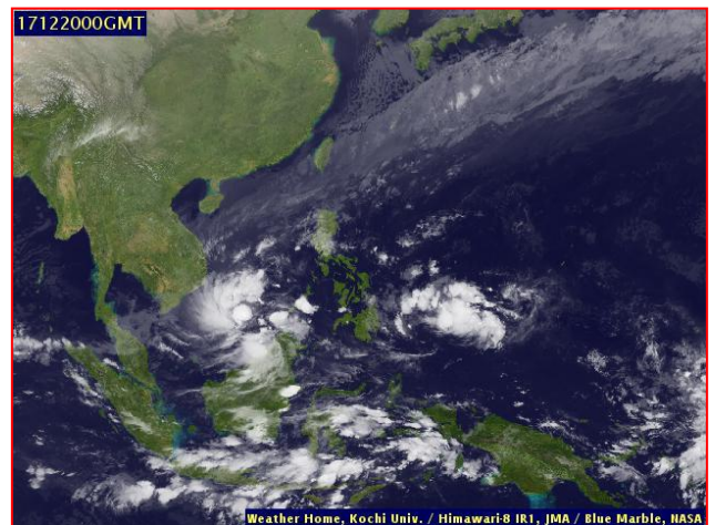
ภาพถ่ายจากดาวเทียม วันที่ ๒๐ ธ.ค. ๒๕๖๐ เวลา ๐๗.๐๐ น.
