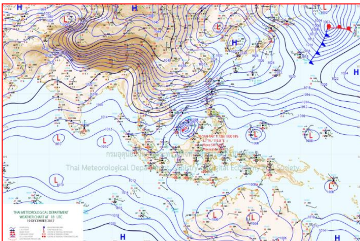
แผนที่อากาศ วันที่ ๒๐ ธ.ค. ๒๕๖๐ เวลา ๐๑.๐๐ น.
