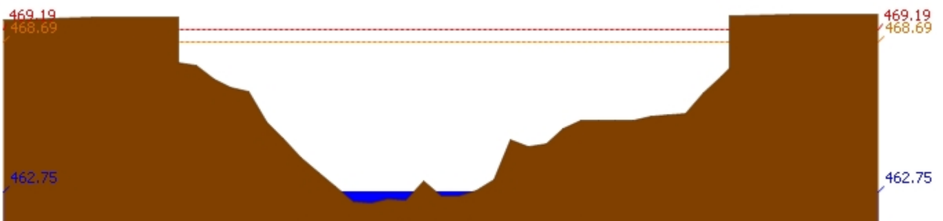
สถานี 060905T น้ำแม่ลี้ที่อำเภอลี้ ต.ลี้ อ.ลี้ จ.ลำพูน ระดับน้ำ 462.75 ม.รทก.
