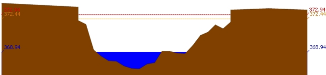
สถานี 060109T แม่น้ำปิงที่บ้านสบอ้อ ต.แม่่นะ อ.เชียงดาว จ.เชียงใหม่ ระดับน้ำ 368.94 ม.รทก.
