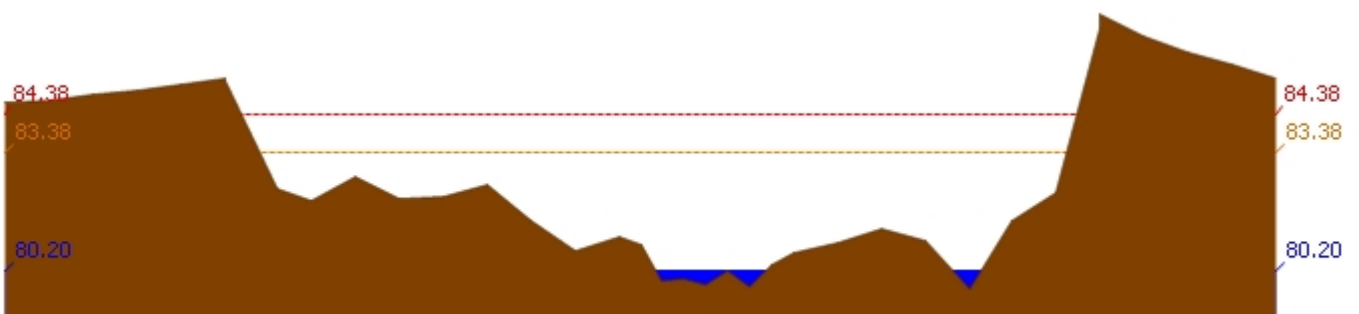
สถานี 062001T คลองสวนหมากที่บ้านน้ำไทรง ต.ท่าขุนราม อ.เมือง จ.กำแพงเพชร ระดับน้ำ 80.20 ม.รทก.
