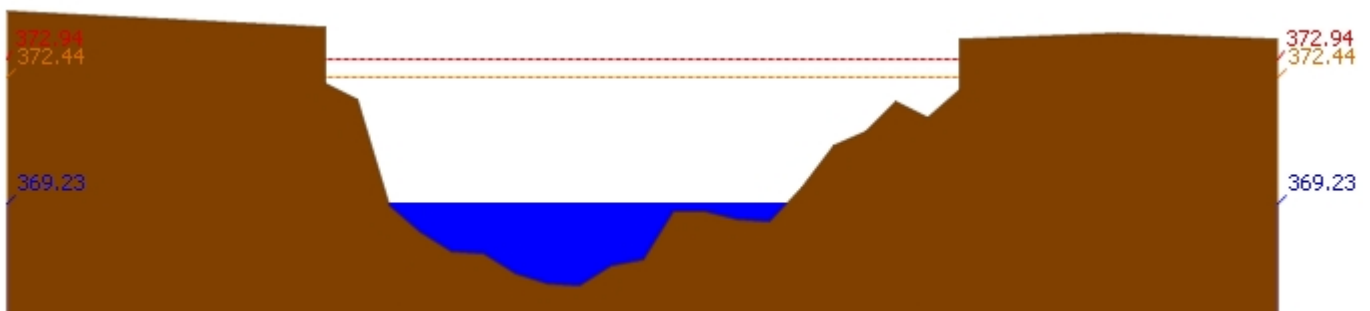
สถานี 060109T แม่น้ำปิงที่บ้านสบอ้อ ต.แม่่นะ อ.เชียงดาว จ.เชียงใหม่ ระดับน้ำ 369.23 ม.รทก.
