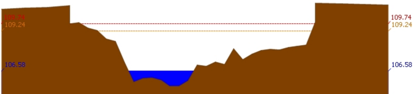
สถานี 061701T ห้วยแม่ท้อที่อำเภอเมืองตาก ต.แม่ท้อ อ.เมืองตาก จ.ตาก ระดับน้ำ 106.58 ม.รทก.
