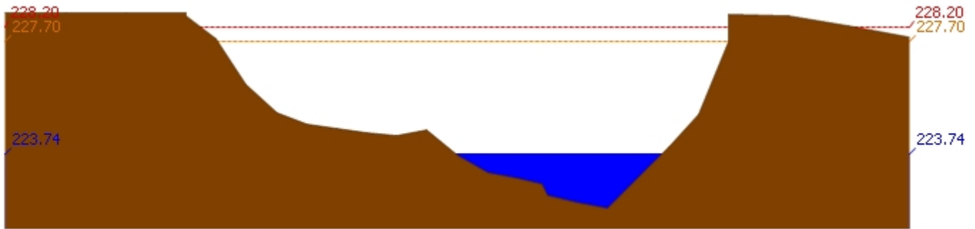
สถานี 070703T น้ำแม่คำที่บ้านนาบอน ต.ทุ่งงาม อ.เสริมงาม จ.ลำปาง ระดับน้ำ 223.74 ม.รทก.
