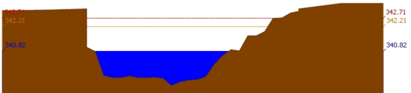
สถานี 070304T น้ำแม่สอยที่บ้านหนองกอก ต.แม่สอก อ.แจ้ห่ม จ.ลำปาง ระดับน้ำ 340.82 ม.รทก.
