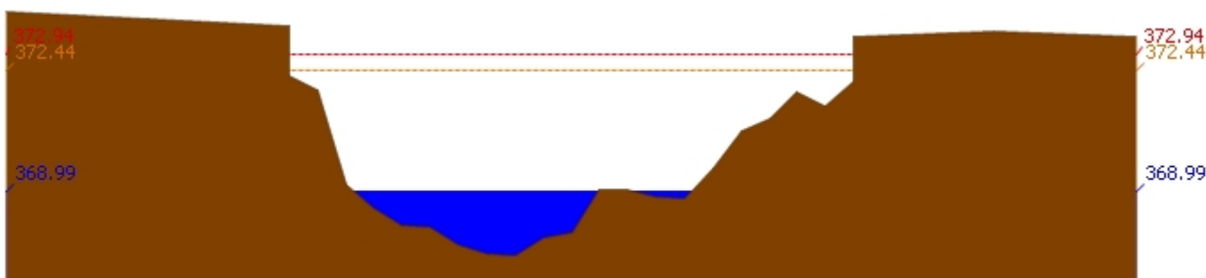
สถานี 060109T แม่น้ำปิงที่บ้านสบอ้อ ต.แม่ระ อ.เชียงดาว จ.เชียงใหม่ ระดับน้ำ 368.99 ม.รทก.
