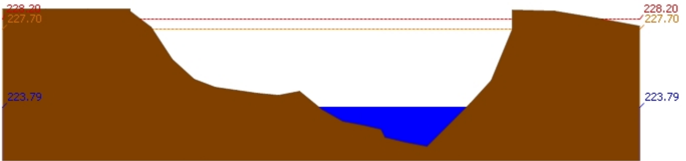
สถานี 070703T น้ำแม่ตำที่บ้านนาบอน ต.ทุ่งงาม อ.เสริมงาม จ.ลำปาง ระดับน้ำ 223.79 ม.รทก.
