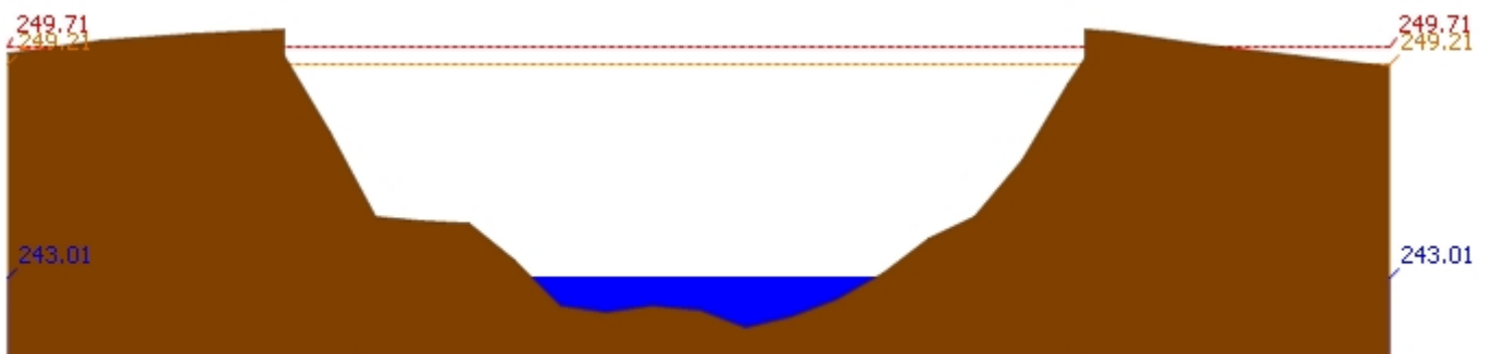
สถานี 070112T แม่น้ำวังที่บ้านบุญนาศ ต.บุญนาศพัฒนา อ.เมืองลำปาง จ.ลำปาง ระดับน้ำ 243.01 ม.รทก.
