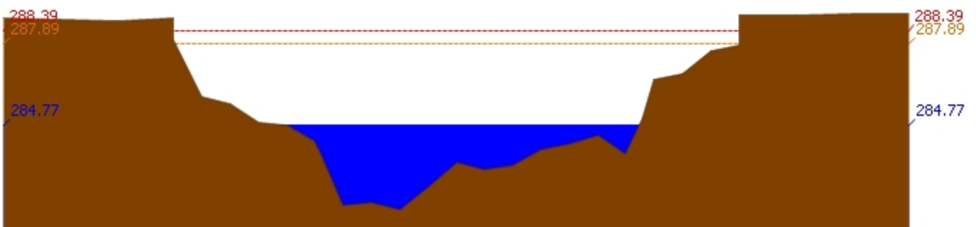
สถานี 070111T แม่น้ำวังที่บ้านเป็นโป่งชัย ต.บ้านเสา อ.แจ้ห่ม จ.ลำปาง ระดับน้ำ 284.77 ม.รทก.
