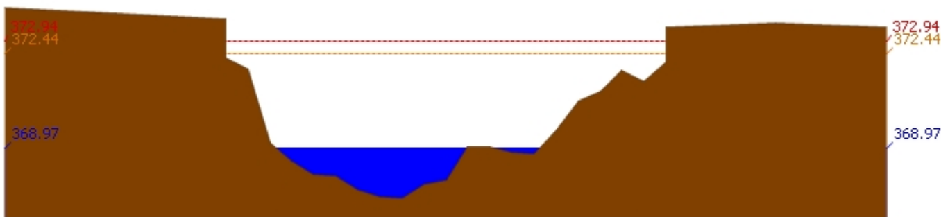
สถานี 060109T แม่น้ำปิงที่บ้านสบอ้อ ต.แม่ระ อ.เชียงดาว จ.เชียงใหม่ ระดับน้ำ 368.97 ม.รทก.
