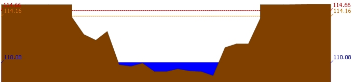
สถานี 061801T คลองวังเจ้าที่บ้านคลองลึก ต.เชียงทอง อ.วังเจ้า จ.ตาก ระดับน้ำ 110.08 ม.รทก.
