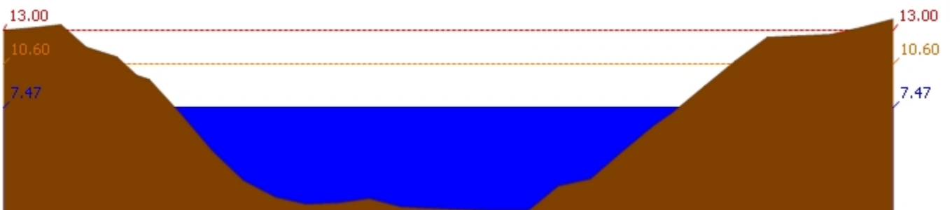
สถานี 120106T แม่น้ำป่าสักที่ อ.เสนาห์ ต.ศาลาวิไทย อ.เสนาห์ จ.สระบุรี ระดับน้ำ 7.47 ม.รทก.
