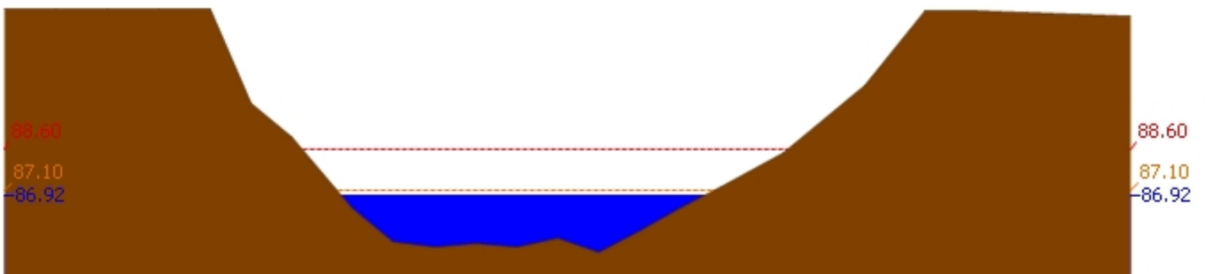
สถานี 120110T แม่น้ำป่าสักที่บ้านวังโบสถ์ ต.วังโบสถ์ อ.หนองไผ่ จ.เพชรบูรณ์ ระดับน้ำ 86.92 ม.รทก.
