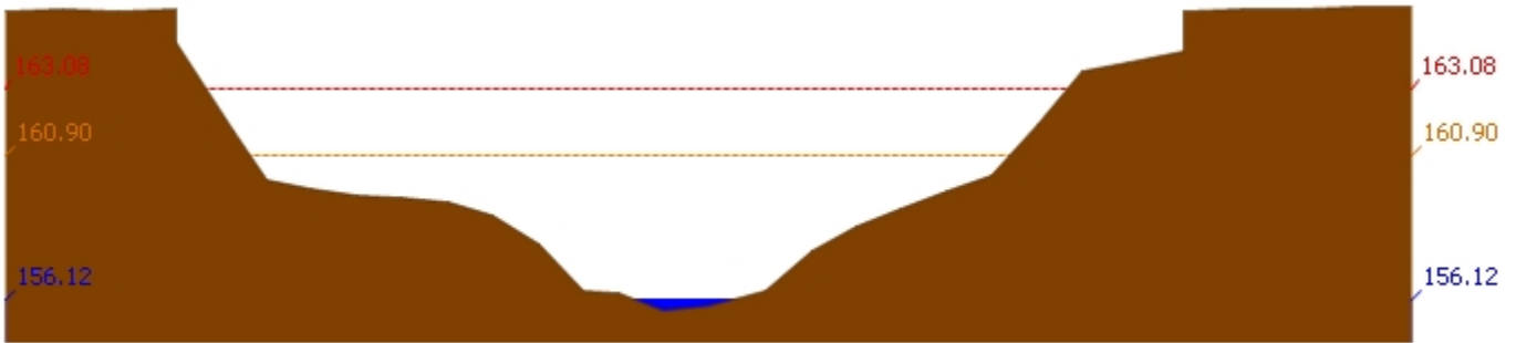
สถานี 120105T แม่น้ำป่าสักที่บ้านวังมเสหนือ ต.ทำอัญญ อ.หล่มสัก จ.เพชรบูรณ์ ระดับน้ำ 156.12 ม.รทก.
