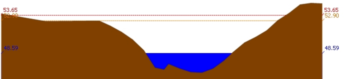
สถานี 120113T แม่น้ำป่าสักที่บ้านเขาค้าง ต.คลองกระจิง อ.ศรีเทพ จ.เพชรบูรณ์ ระดับน้ำ 48.59 ม.รทก.
