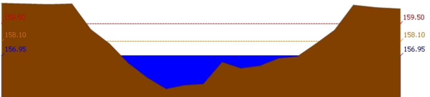
สถานี 120305T หัวน้ำพุที่ อ.หล่มเก่า ต.หล่มเก่า อ.หล่มเก่า จ.เพชรบูรณ์ ระดับน้ำ 156.95 ม.รทก.
