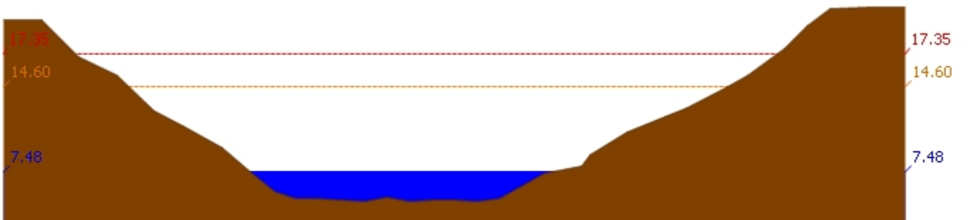
สถานี 120109T แม่น้ำป่าสักที่ อ.แก่งคอย ต.แก่งคอย อ.แก่งคอย จ.สระบุรี ระดับน้ำ 7.48 ม.รทก.
