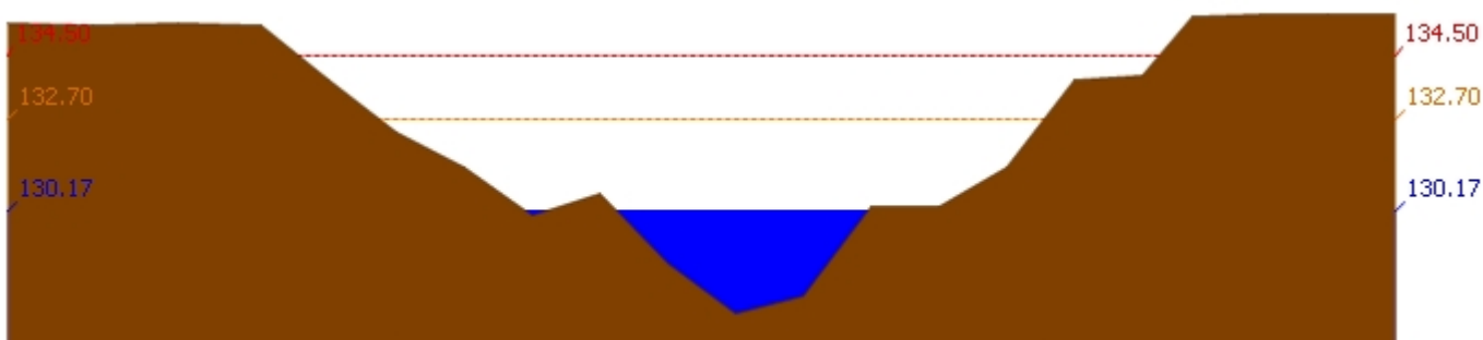
สถานี 120111T แม่น้ำป่าสักที่บ้านจางวาง ต.ลานบัว อ.หล่มสัก จ.เพชรบูรณ์ ระดับน้ำ 130.17 ม.รทก.
