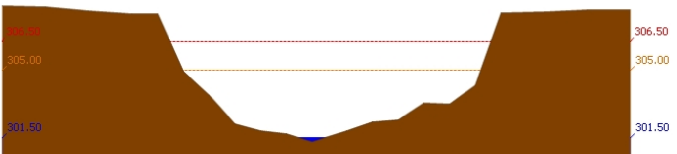
สถานี 120304T หัวน้ำพุที่บ้านกกกะบาก ต.โป่ง อ.ด่านซ้าย จ.เลย ระดับน้ำ 301.50 ม.รทก.
