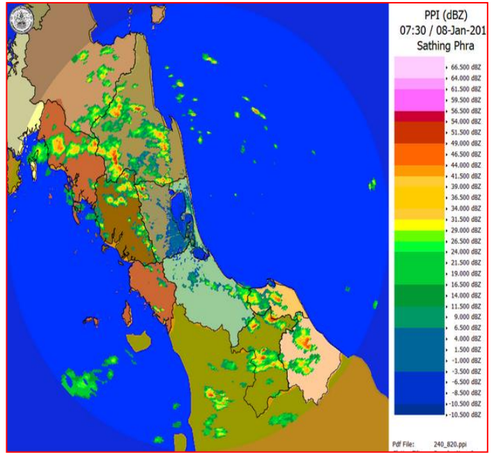
สถานีสีหิงพระ เวลา ๑๔.๓๐ น.
