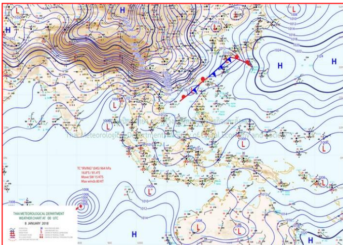
แผนที่อากาศ วันที่ ๘ ม.ค. ๒๕๖๑ เวลา ๐๗.๐๐ น.
