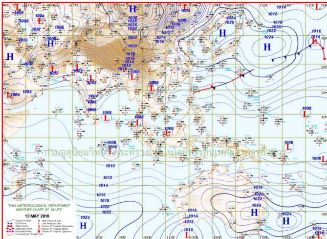
แผนที่อากาศ วันที่ ๑๔ พ.ค. ๒๕๕๙ เวลา ๐๑.๐๐ น.
