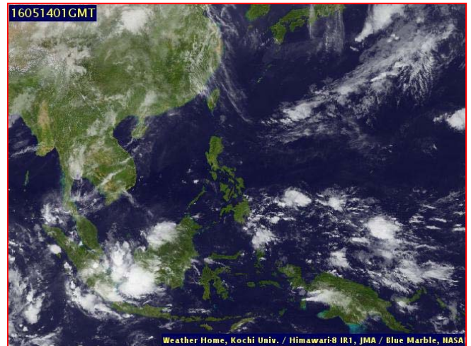
ภาพถ่ายจากดาวเทียม วันที่ ๑๔ พ.ค. ๒๕๕๙ เวลา ๐๘.๐๐ น.
