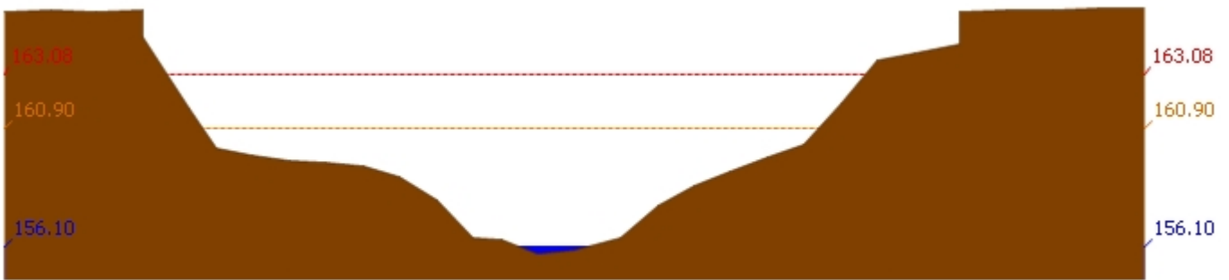
สถานี 120105T แม่น้ำป่าสักที่บ้านวังมเสหนือ ต.ทำอัญญ อ.หล่มสัก จ.เพชรบูรณ์ ระดับน้ำ 156.10 ม.รทก.
