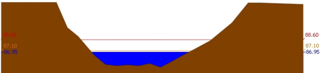
สถานี 120110T แม่น้ำป่าสักที่บ้านวังโบสถ์ ต.วังโบสถ์ อ.หนองไผ่ จ.เพชรบูรณ์ ระดับน้ำ 86.95 ม.รทก.
