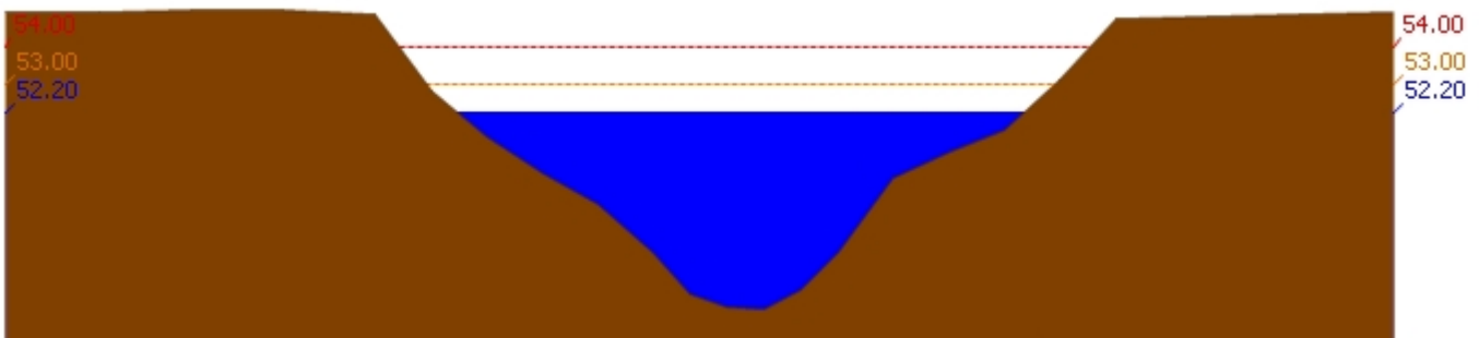
สถานี 120702T ลำสนธิที่บ้านท่าช้าง ต.หนองขาหย่าง อ.ชัยบาดาล จ.ลพบุรี ระดับน้ำ 52.20 ม.รทก.
