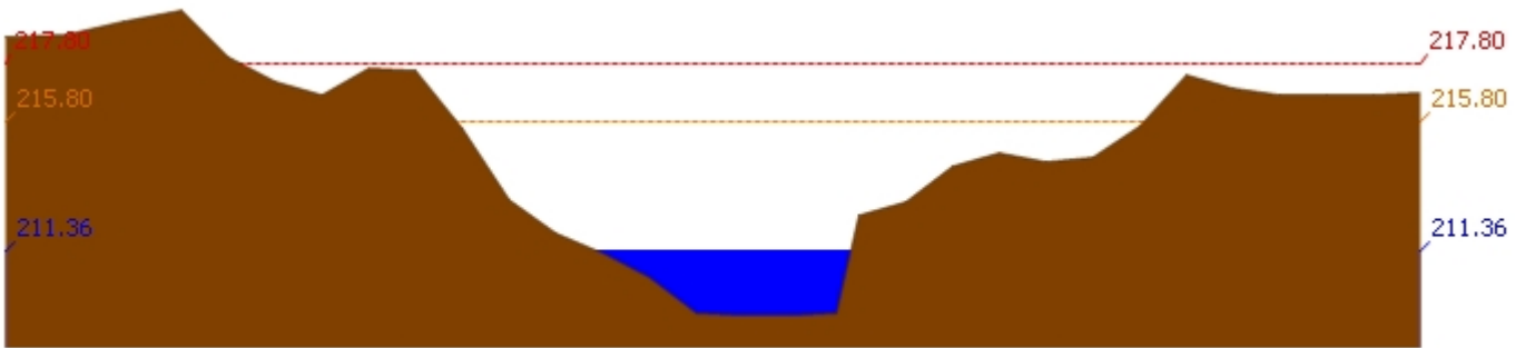
สถานี 120205T แม่น้ำป่าสักที่บ้านอู่กระทัด ต.ศิลา อ.หล่มเก่า จ.เพชรบูรณ์ ระดับน้ำ 211.36 ม.รทก.
