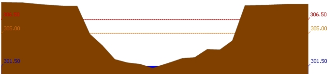
สถานี 120304T ห้วยน้ำพุที่บ้านกกกะบาก ต.โป่ง อ.ด่านซ้าย จ.เลย ระดับน้ำ 301.50 ม.รทก.
