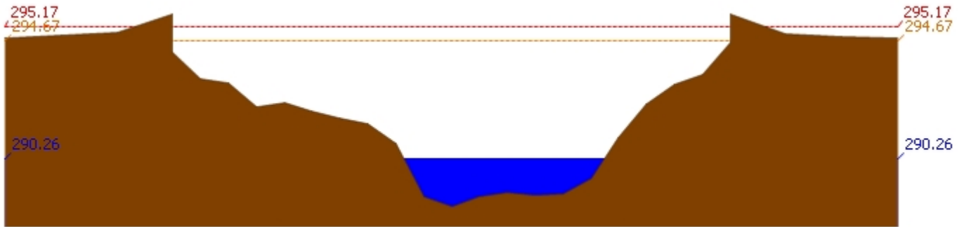
สถานี 060709T น้ำแม่กวังที่ลำพูน ต.เวียงของ อ.เมือง จ.ลำพูน ระดับน้ำ 290.26 ม.รทก.
