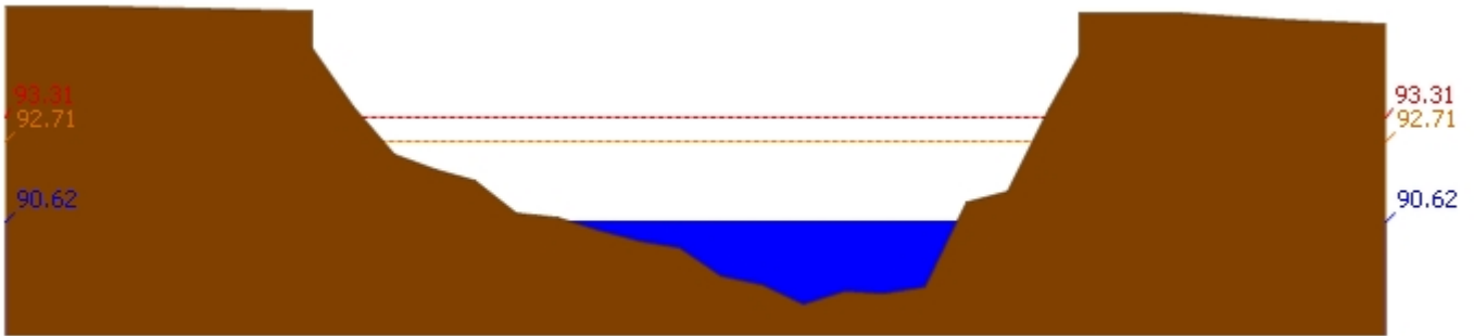
สถานี 061901T คลองแม่ระกาที่บ้านวังชะโอน ต.ท่าไม้ อ.พรานกระต่าย จ.กำแพงเพชร ระดับน้ำ 90.62 ม.รทก.
