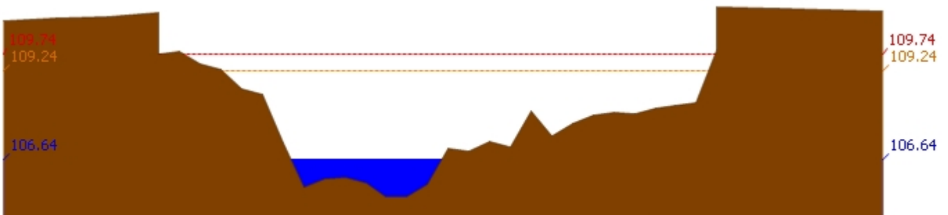
สถานี 061701T ห้วยแม่ท้อที่อำเภอเมืองตาก ต.แม่ท้อ อ.เมืองตาก จ.ตาก ระดับน้ำ 106.64 ม.รทก.
