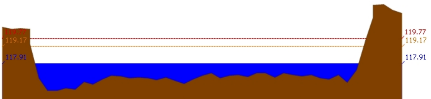
สถานี 060111T แม่น้ำปิงที่บ้านปากร่องห้วยจี่ ต.ตากออก อ.บ้านตาก จ.ตาก ระดับน้ำ 117.91 ม.รทก.
