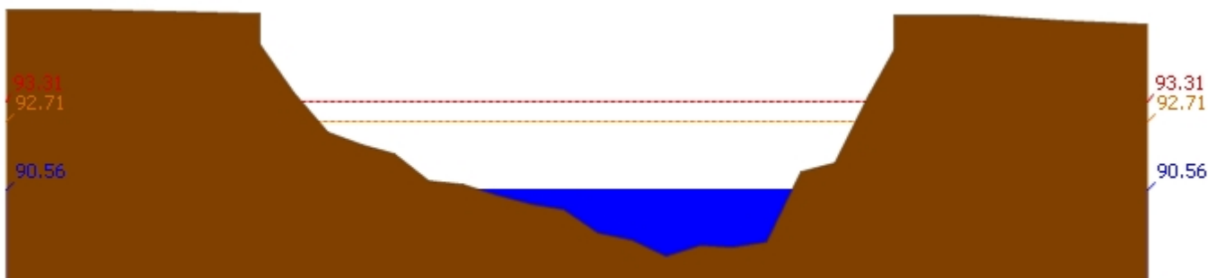
สถานี 061901T คลองแม่ระกาที่บ้านวังชะโอน ต.ท่าไม้ อ.พรานกระต่าย จ.กำแพงเพชร ระดับน้ำ 90.56 ม.รทก.
