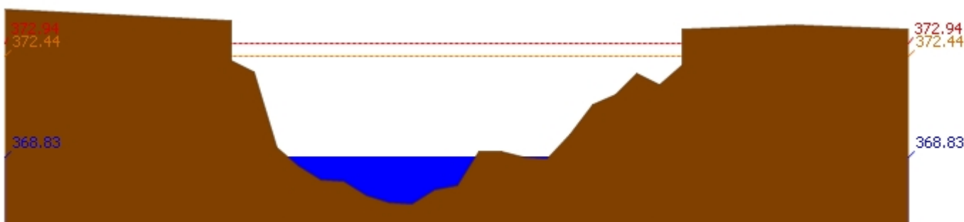
สถานี 060109T แม่น้ำปิงที่บ้านสบอ้อ ต.แม่่นะ อ.เชียงดาว จ.เชียงใหม่ ระดับน้ำ 368.83 ม.รทก.
