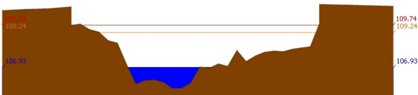
สถานี 061701T ห้วยแม่ท้อที่อำเภอเมืองตาก ต.แม่ท้อ อ.เมืองตาก จ.ตาก ระดับน้ำ 106.93 ม.รทก.
