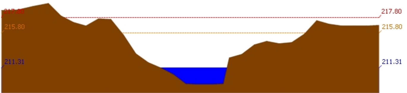
สถานี 120205T แม่น้ำป่าสักที่บ้านอู่กะทาด ต.ศิลา อ.หล่มเก่า จ.เพชรบูรณ์ ระดับน้ำ 211.31 ม.รทก.
