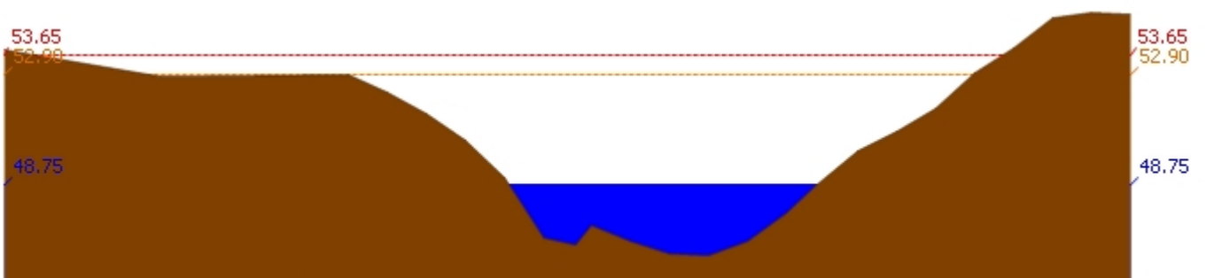
สถานี 120113T แม่น้ำป่าสักที่บ้านเขาค้าง ต.คลองกระจิง อ.ศรีเทพ จ.เพชรบูรณ์ ระดับน้ำ 48.75 ม.รทก.
