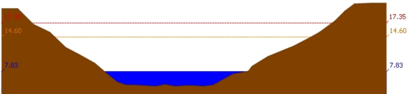
สถานี 120109T แม่น้ำป่าสักที่ อ.แก่งคอย ต.แก่งคอย อ.แก่งคอย จ.สระบุรี ระดับน้ำ 7.83 ม.รทก.
