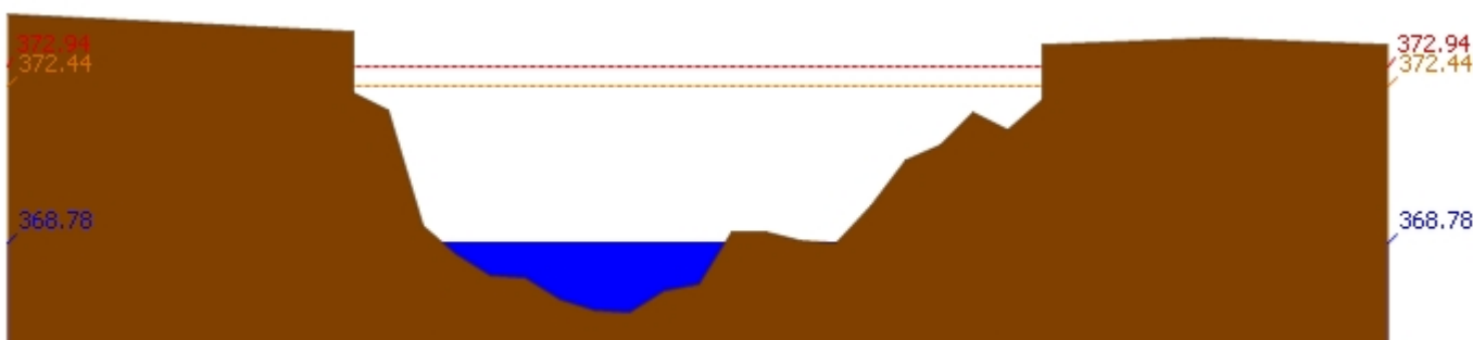
สถานี 060109T แม่น้ำปิงที่บ้านสบอ้อ ต.แม่่นะ อ.เชียงดาว จ.เชียงใหม่ ระดับน้ำ 368.78 ม.รทก.
