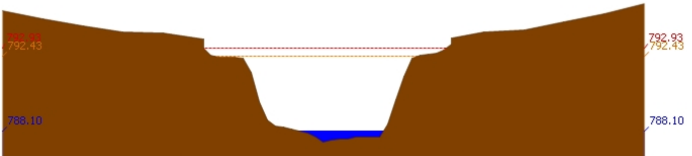
สถานี 061503T น้ำแม่ต้นที่บ้านคอย ต.ยางเปียง อ.อมก๋อย จ.เชียงใหม่ ระดับน้ำ 788.10 ม.รทก.
