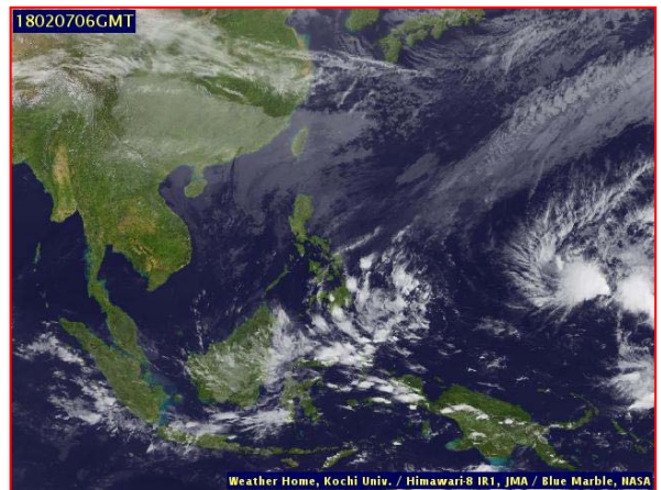
ภาพถ่ายจากดาวเทียม วันที่ ๗ ก.พ. ๒๕๖๑ เวลา ๑๓.๐๐ น.
