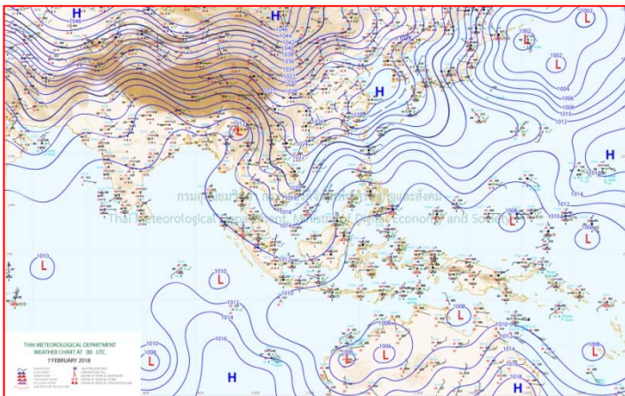
แผนที่อากาศ วันที่ ๗ ก.พ. ๒๕๖๑ เวลา ๐๗.๐๐ น.
