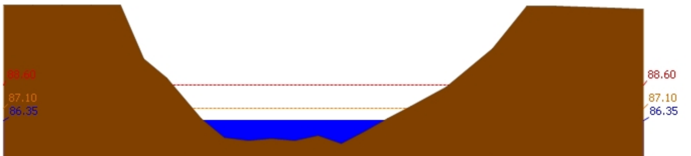
สถานี 120110T แม่น้ำป่าสักที่บ้านวังโบสถ์ ต.วังโบสถ์ อ.หนองไผ่ จ.เพชรบูรณ์ ระดับน้ำ 86.35 ม.รทก.
