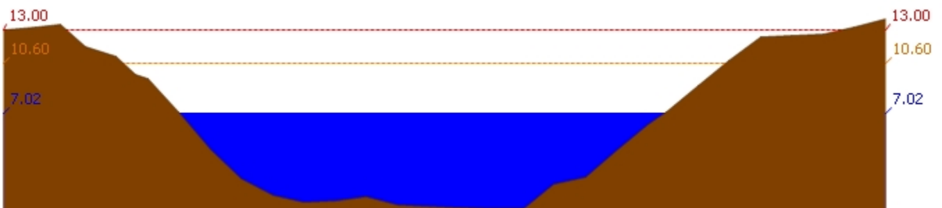
สถานี 120106T แม่น้ำป่าสักที่ อ.เสนาห์ ต.ศาลาวิไทย อ.เสนาห์ จ.สระบุรี ระดับน้ำ 7.02 ม.รทก.
