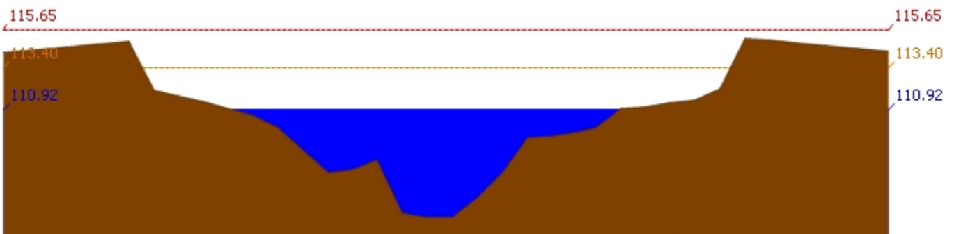
สถานี 120107T แม่น้ำป่าสักที่ อ.เมืองเพชรบูรณ์ ต.นาป่า อ.เมือง จ.เพชรบูรณ์ ระดับน้ำ 110.92 ม.รทก.
