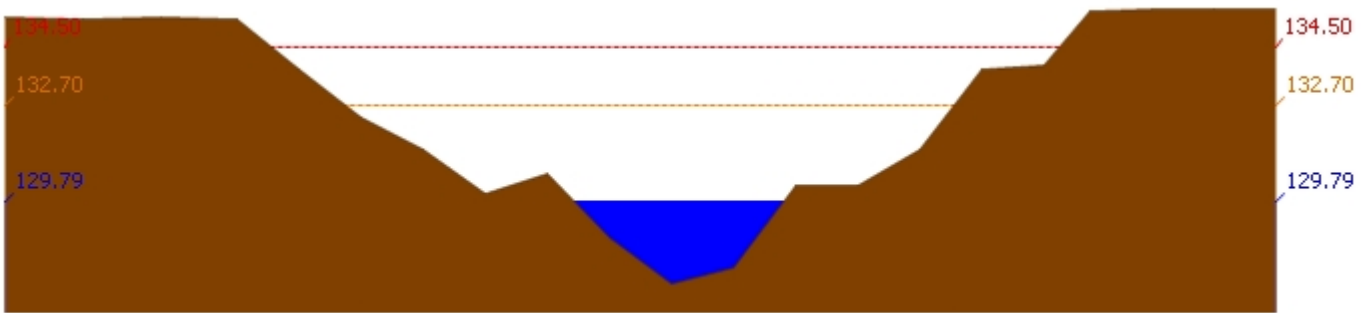
สถานี 120111T แม่น้ำป่าสักที่บ้านจางวาง ต.ลานบัว อ.หล่มสัก จ.เพชรบูรณ์ ระดับน้ำ 129.79 ม.รทก.
