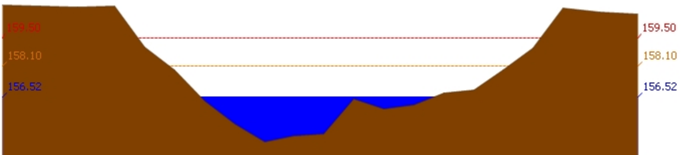
สถานี 120305T หัวน้ำพุที่ อ.หล่มเก่า ต.หล่มเก่า อ.หล่มเก่า จ.เพชรบูรณ์ ระดับน้ำ 156.52 ม.รทก.
