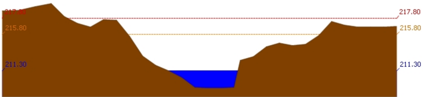
สถานี 120205T แม่น้ำป่าสักที่บ้านอู่กะทาด ต.ศิลา อ.หล่มเก่า จ.เพชรบูรณ์ ระดับน้ำ 211.30 ม.รทก.
