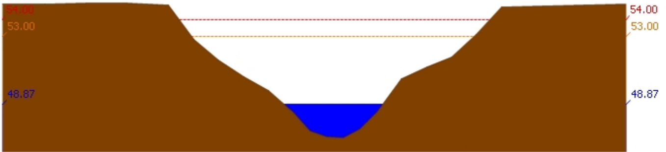
สถานี 120702T ลำสนธิที่บ้านท่าช้าง ต.หนองขาหย่าง อ.ชัยบาดาล จ.ลพบุรี ระดับน้ำ 48.87 ม.รทก.
