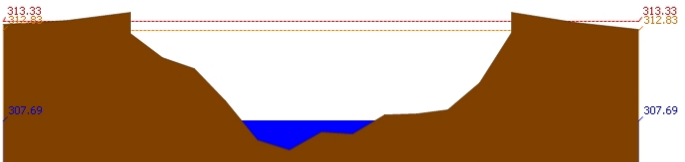
สถานี 060814T น้ำแม่ขานที่บ้านท่าโป่ง ต.บ้านแม อ.สันป่าตอง จ.เชียงใหม่ ระดับน้ำ 307.69 ม.รทก.
