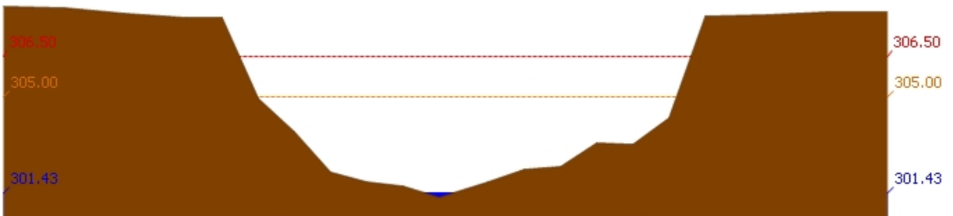
สถานี 120304T ห้วยน้ำพุที่บ้านกกกะบาก ต.โป่ง อ.ด่านซ้าย จ.เลย ระดับน้ำ 301.43 ม.รทก.
