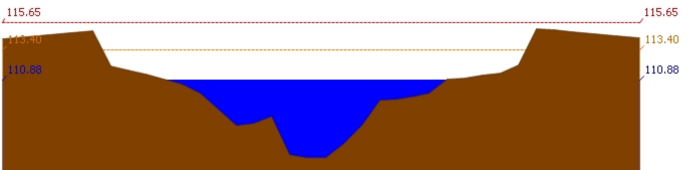
สถานี 120107T แม่น้ำป่าสักที่ อ.เมืองเพชรบูรณ์ ต.นาป่า อ.เมือง จ.เพชรบูรณ์ ระดับน้ำ 110.88 ม.รทก.
