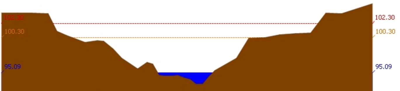
สถานี 120112T แม่น้ำป่าสักที่บ้านหนองแหวน ต.วังมะข่อ อ.เมือง จ.เพชรบูรณ์ ระดับน้ำ 95.09 ม.รทก.
