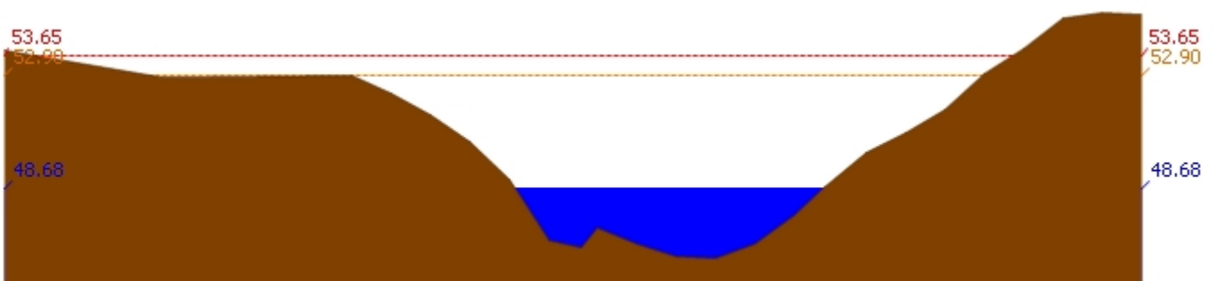
สถานี 120113T แม่น้ำป่าสักที่บ้านเขาค้าง ต.คลองกระจิง อ.ศรีเทพ จ.เพชรบูรณ์ ระดับน้ำ 48.68 ม.รทก.
