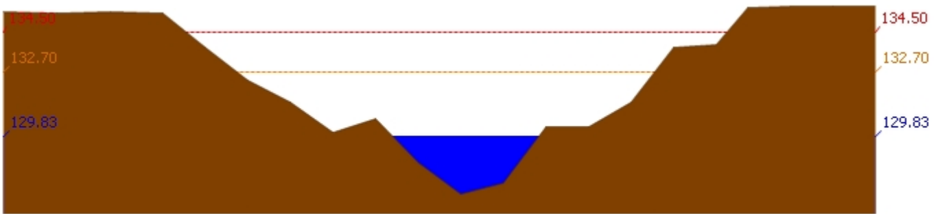
สถานี 120111T แม่น้ำป่าสักที่บ้านจางวาง ต.ลานบัว อ.หล่มสัก จ.เพชรบูรณ์ ระดับน้ำ 129.83 ม.รทก.
