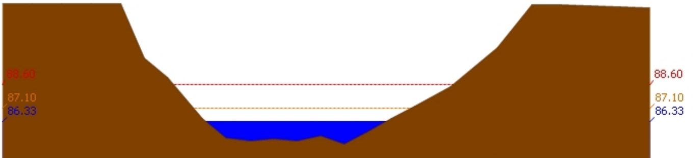
สถานี 120110T แม่น้ำป่าสักที่บ้านวังโบสถ์ ต.วังโบสถ์ อ.หนองไผ่ จ.เพชรบูรณ์ ระดับน้ำ 86.33 ม.รทก.
