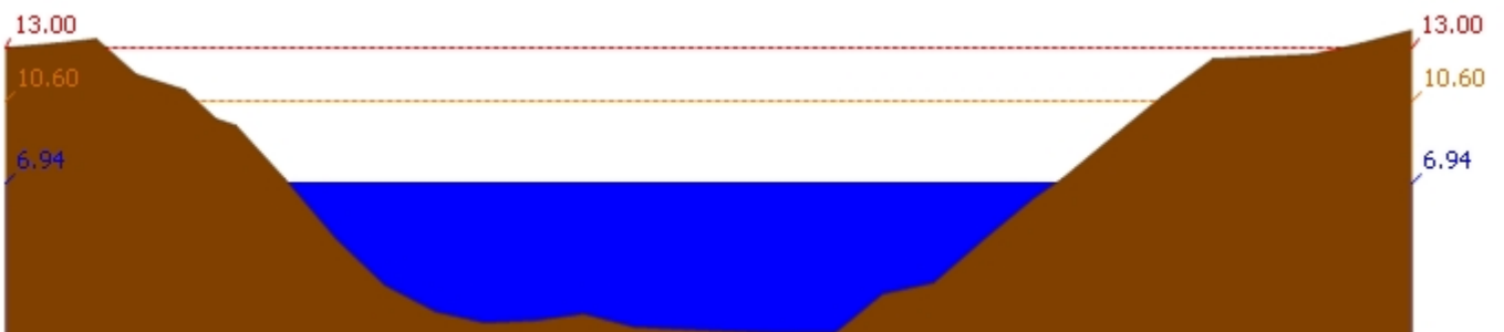
สถานี 120106T แม่น้ำป่าสักที่ อ.เสนาห์ ต.ศาลาวิไทย อ.เสนาห์ จ.สระบุรี ระดับน้ำ 6.94 ม.รทก.
