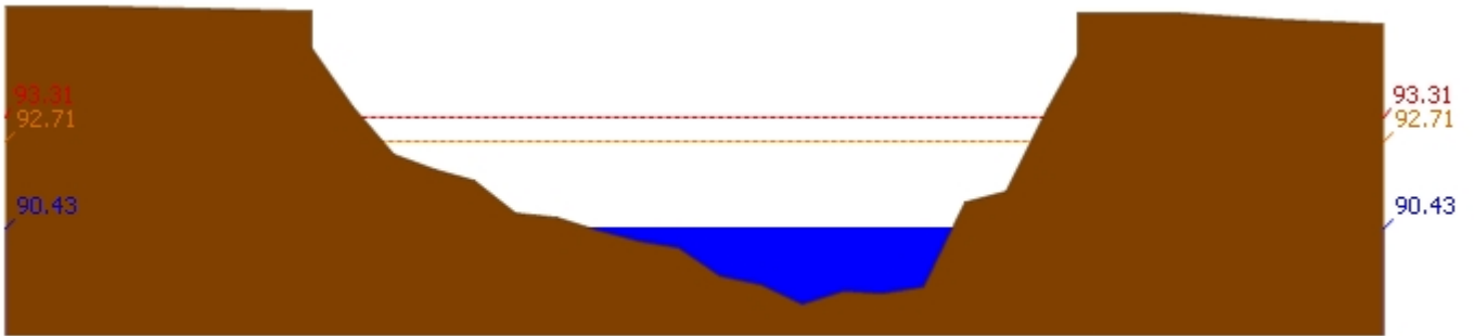
สถานี 061901T คลองแม่ระกาที่บ้านวังชะโอน ต.ท่าไม้ อ.พรานกระต่าย จ.กำแพงเพชร ระดับน้ำ 90.43 ม.รทก.
