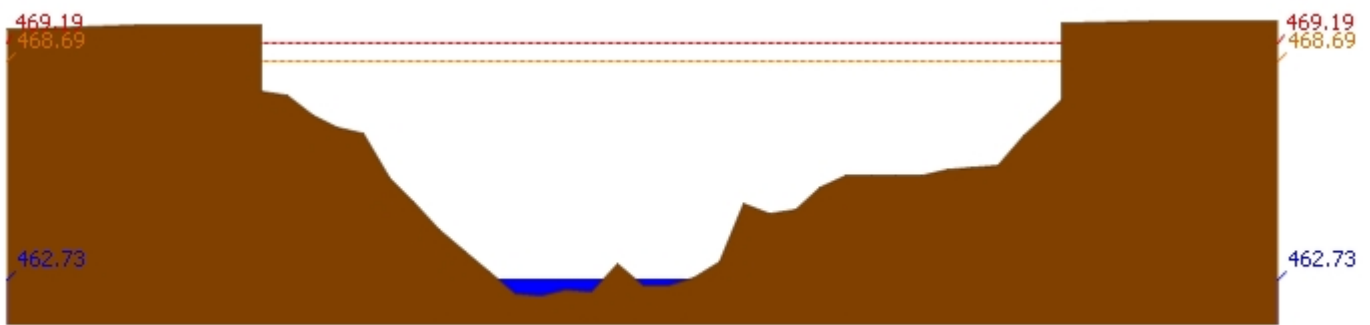
สถานี 060905T น้ำแม่ลีที่อำเภอลี้ ต.ลี อ.ลี จ.ลำพูน ระดับน้ำ 462.73 ม.รทก.
