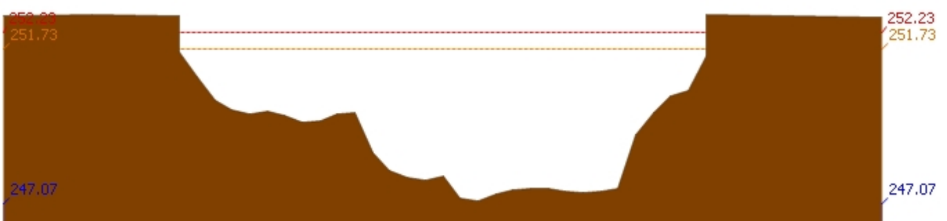
สถานี 070403T น้ำแม่ต๋อยที่บ้านแค ต.บ้านเป้า อ.เมืองลำปาง จ.ลำปาง ระดับน้ำ 247.07 ม.รทก.
