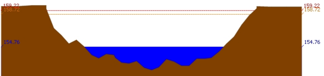
สถานี 070117T แม่น้ำวังที่เทศบาลตำบลแม่ป๋อ ต.แม่ป๋อ อ.แม่พริก จ.ลำปาง ระดับน้ำ 154.76 ม.รทก.
