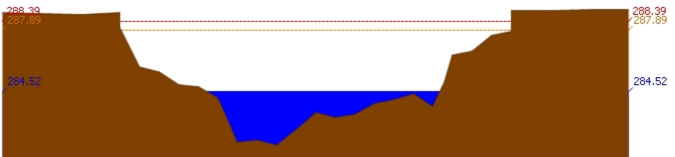
สถานี 070111T แม่น้ำวังที่บ้านโป่งชัย ต.บ้านเสา อ.แจ้ห่ม จ.ลำปาง ระดับน้ำ 284.52 ม.รทก.
