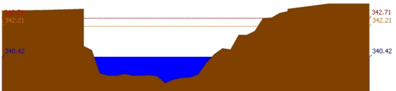
สถานี 070304T น้ำแม่สอยที่บ้านหนองกอก ต.แม่สวก อ.แจ้ห่ม จ.ลำปาง ระดับน้ำ 340.42 ม.รทก.
