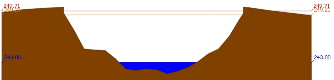
สถานี 070112T แม่น้ำวังที่บ้านบุญนา ต.บุญนาพัฒนา อ.เมืองลำปาง จ.ลำปาง ระดับน้ำ 243.00 ม.รทก.
