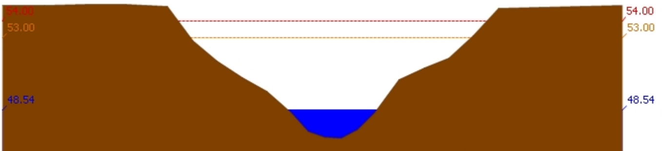
สถานี 120702T ลำสนธิที่บ้านท่าช้าง ต.หนองขาหย่าง อ.ชัยบาดาล จ.ลพบุรี ระดับน้ำ 48.54 ม.รทก.
