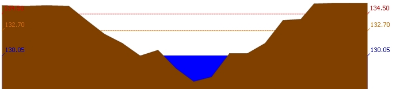
สถานี 120111T แม่น้ำป่าสักที่บ้านจางวาง ต.ลานบัว อ.หล่มสัก จ.เพชรบูรณ์ ระดับน้ำ 130.05 ม.รทก.
