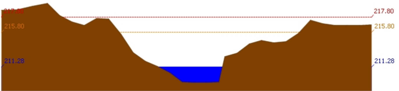
สถานี 120205T แม่น้ำป่าสักที่บ้านอู่กะทาด ต.ศิลา อ.หล่มเก่า จ.เพชรบูรณ์ ระดับน้ำ 211.28 ม.รทก.
