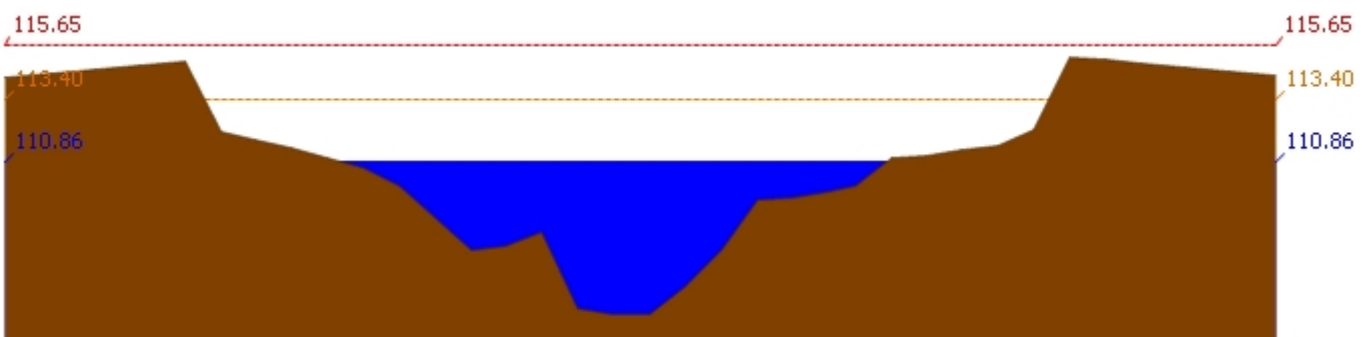
สถานี 120107T แม่น้ำป่าสักที่ อ.เมืองเพชรบูรณ์ ต.นาป่า อ.เมือง จ.เพชรบูรณ์ ระดับน้ำ 110.86 ม.รทก.
