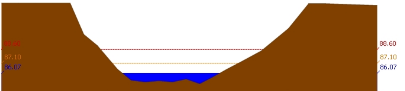
สถานี 120110T แม่น้ำป่าสักที่บ้านวังโบสถ์ ต.วังโบสถ์ อ.หนองไผ่ จ.เพชรบูรณ์ ระดับน้ำ 86.07 ม.รทก.
