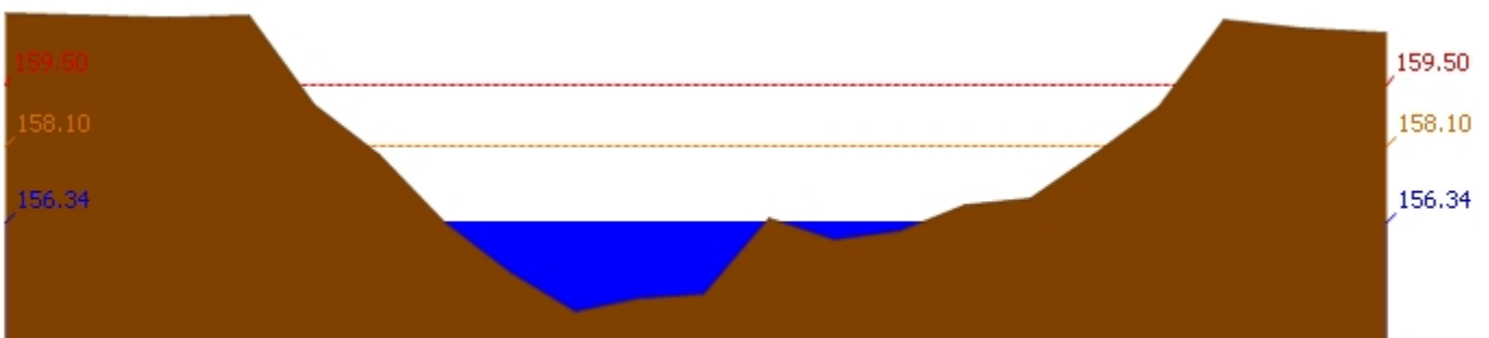
สถานี 120305T หัวเขื่อนที่ อ.หล่มเก่า ต.หล่มเก่า อ.หล่มเก่า จ.เพชรบูรณ์ ระดับน้ำ 156.34 ม.รทก.
