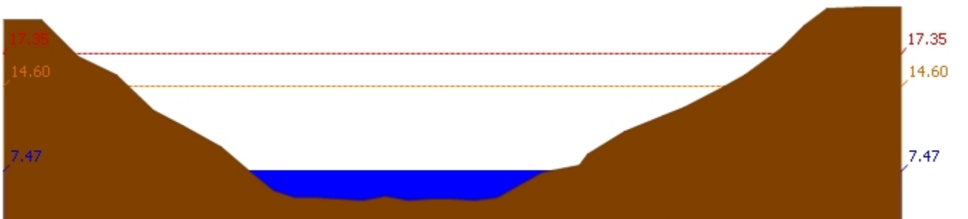
สถานี 120109T แม่น้ำป่าสักที่ อ.แก่งคอย ต.แก่งคอย อ.แก่งคอย จ.สระบุรี ระดับน้ำ 7.47 ม.รทก.
