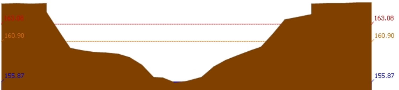
สถานี 120105T แม่น้ำป่าสักที่บ้านวังมเสหนือ ต.ทำอัญญ อ.หล่มสัก จ.เพชรบูรณ์ ระดับน้ำ 155.87 ม.รทก.
