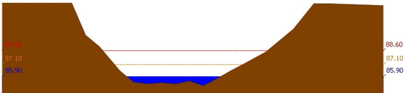
สถานี 120110T แม่น้ำป่าสักที่บ้านวังโบสถ์ ต.วังโบสถ์ อ.หนองไผ่ จ.เพชรบูรณ์ ระดับน้ำ 85.90 ม.รทก.
