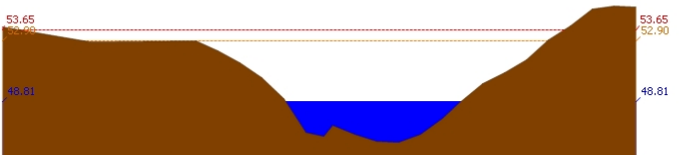
สถานี 120113T แม่น้ำป่าสักที่บ้านเขาค้าง ต.คลองกระจิง อ.ศรีเทพ จ.เพชรบูรณ์ ระดับน้ำ 48.81 ม.รทก.
