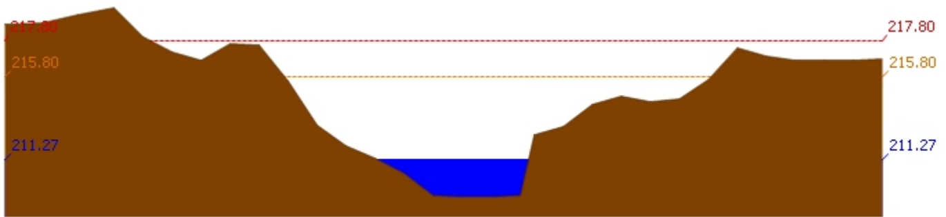
สถานี 120205T แม่น้ำป่าสักที่บ้านอู่กะทาด ต.ศิลา อ.หล่มเก่า จ.เพชรบูรณ์ ระดับน้ำ 211.27 ม.รทก.
