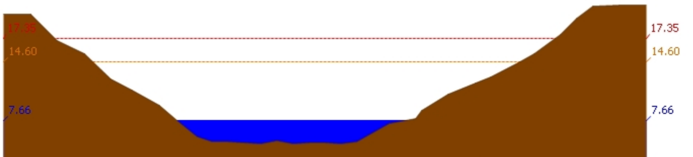
สถานี 120109T แม่น้ำป่าสักที่ อ.แก่งคอย ต.แก่งคอย อ.แก่งคอย จ.สระบุรี ระดับน้ำ 7.66 ม.รทก.
