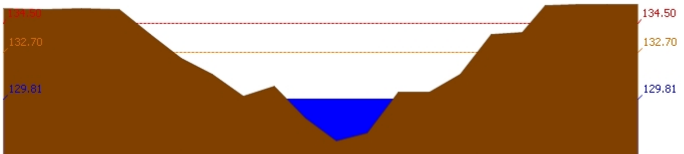
สถานี 120111T แม่น้ำป่าสักที่บ้านจางวาง ต.ลานบัว อ.หล่มสัก จ.เพชรบูรณ์ ระดับน้ำ 129.81 ม.รทก.
