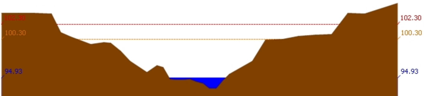
สถานี 120112T แม่น้ำป่าสักที่บ้านหนองแหวน ต.วังมะข่อ อ.เมือง จ.เพชรบูรณ์ ระดับน้ำ 94.93 ม.รทก.
