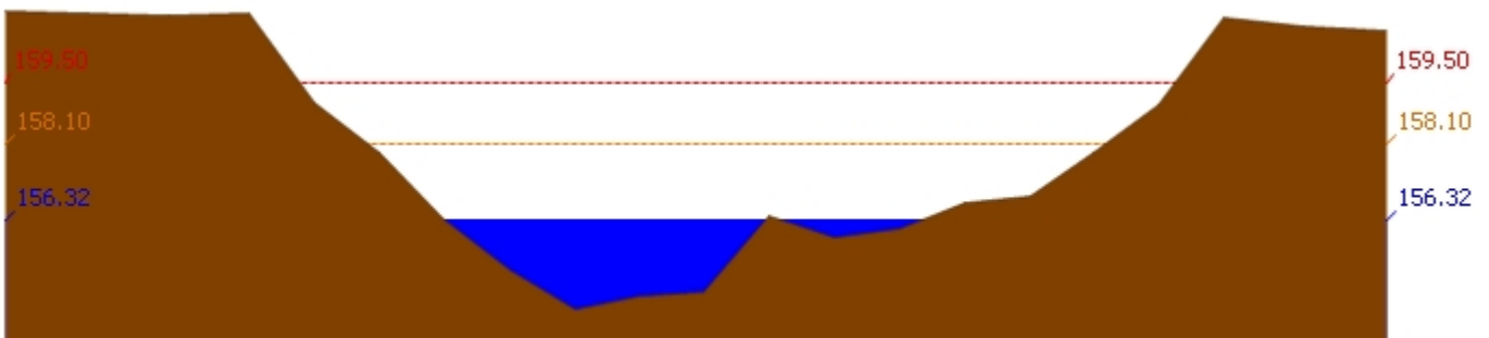
สถานี 120305T หัวน้ำพุที่ อ.หล่มเก่า ต.หล่มเก่า อ.หล่มเก่า จ.เพชรบูรณ์ ระดับน้ำ 156.32 ม.รทก.
