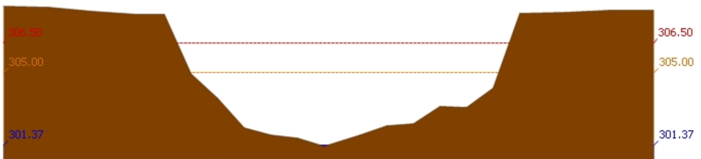
สถานี 120304T ห้วยน้ำพุที่บ้านกกกะบาก ต.โป่ง อ.ด่านซ้าย จ.เลย ระดับน้ำ 301.37 ม.รทก.
