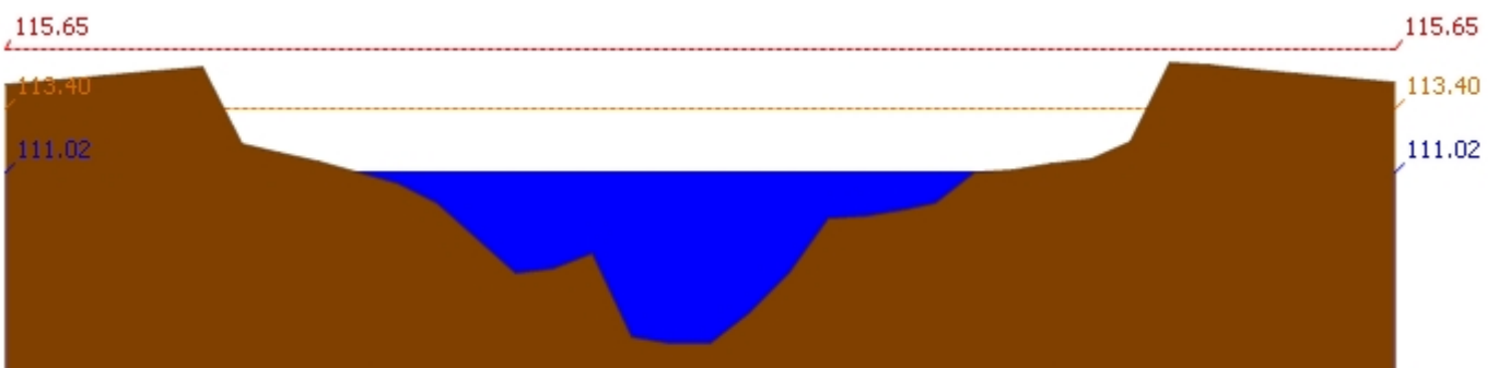
สถานี 120107T แม่น้ำป่าสักที่ อ.เมืองเพชรบูรณ์ ต.นาป่า อ.เมือง จ.เพชรบูรณ์ ระดับน้ำ 111.02 ม.รทก.
