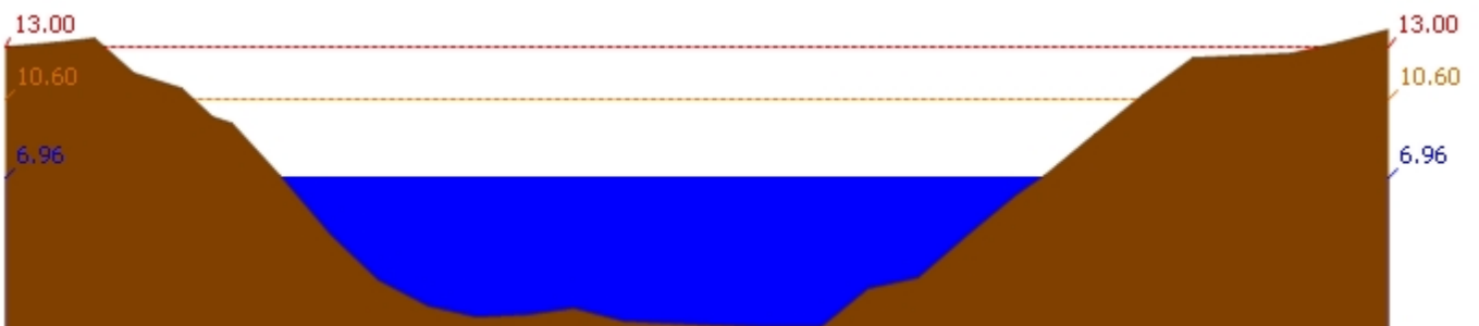
สถานี 120106T แม่น้ำป่าสักที่ อ.เสนาห์ ต.ศาลาวิไทย อ.เสนาห์ จ.สระบุรี ระดับน้ำ 6.96 ม.รทก.
