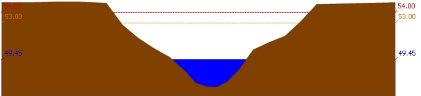
สถานี 120702T ลำสนธิที่บ้านท่าช้าง ต.หนองขาหย่าง อ.ชัยบาดาล จ.ลพบุรี ระดับน้ำ 49.45 ม.รทก.
