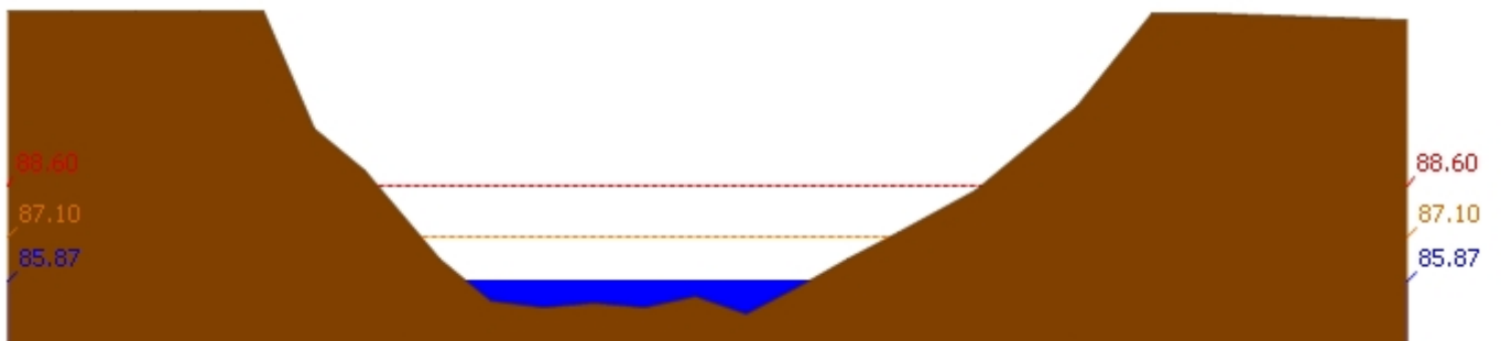
สถานี 120110T แม่น้ำป่าสักที่บ้านวังโบสถ์ ต.วังโบสถ์ อ.หนองไผ่ จ.เพชรบูรณ์ ระดับน้ำ 85.87 ม.รทก.
