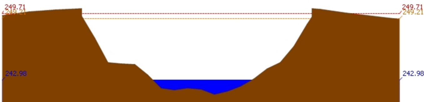
สถานี 070112T แม่น้ำวังที่บ้านบุญนาศ ต.บุญนาศพัฒนา อ.เมืองลำปาง จ.ลำปาง ระดับน้ำ 242.98 ม.รทก.
