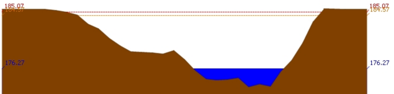
สถานี 070116T แม่น้ำวังที่บ้านแม่เตี๊ยะ ต.แม่ถอด อ.เถิน จ.ลำปาง ระดับน้ำ 176.27 ม.รทก.
