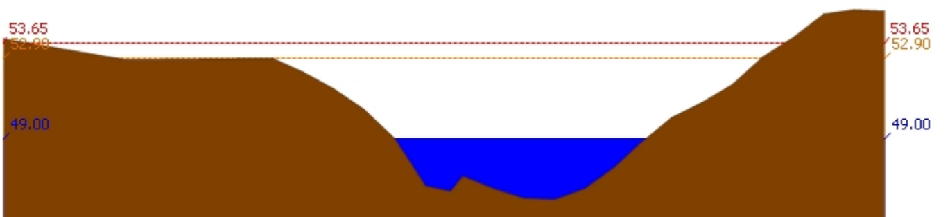
สถานี 120113T แม่น้ำป่าสักที่บ้านเขาค้าง ต.คลองกระจิง อ.ศรีเทพ จ.เพชรบูรณ์ ระดับน้ำ 49.00 ม.รทก.
