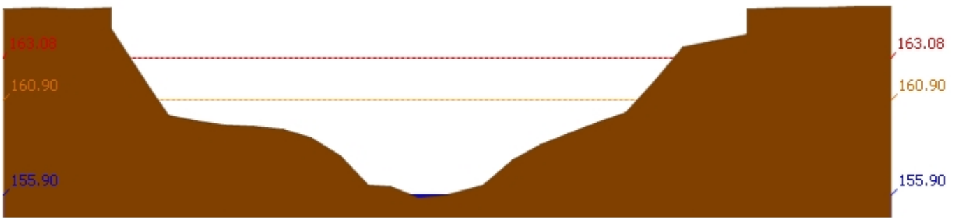
สถานี 120105T แม่น้ำป่าสักที่บ้านวังมเสเหนือ ต.ทำอิบุญ อ.หล่มสัก จ.เพชรบูรณ์ ระดับน้ำ 155.90 ม.รทก.
