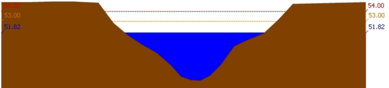
สถานี 120702T ลำสนธิที่บ้านท่าช้าง ต.หนองขาหย่าง อ.ชัยบาดาล จ.ลพบุรี ระดับน้ำ 51.82 ม.รทก.
