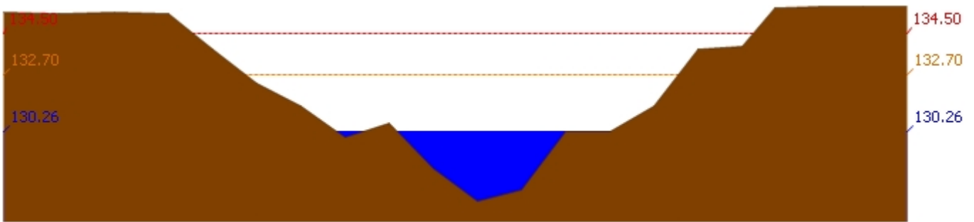
สถานี 120111T แม่น้ำป่าสักที่บ้านจางวาง ต.ลานบัว อ.หล่มสัก จ.เพชรบูรณ์ ระดับน้ำ 130.26 ม.รทก.
