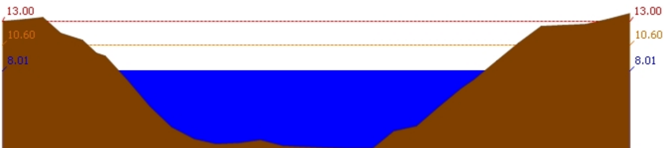
สถานี 120106T แม่น้ำป่าสักที่ อ.เสนาห์ ต.ศาลาวิไทย อ.เสนาห์ จ.สระบุรี ระดับน้ำ 8.01 ม.รทก.
