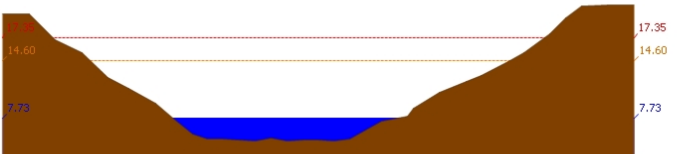
สถานี 120109T แม่น้ำป่าสักที่ อ.แก่งคอย ต.แก่งคอย อ.แก่งคอย จ.สระบุรี ระดับน้ำ 7.73 ม.รทก.
