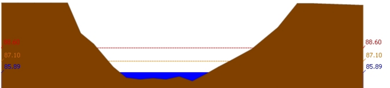
สถานี 120110T แม่น้ำป่าสักที่บ้านวังโบสถ์ ต.วังโบสถ์ อ.หนองไผ่ จ.เพชรบูรณ์ ระดับน้ำ 85.89 ม.รทก.
