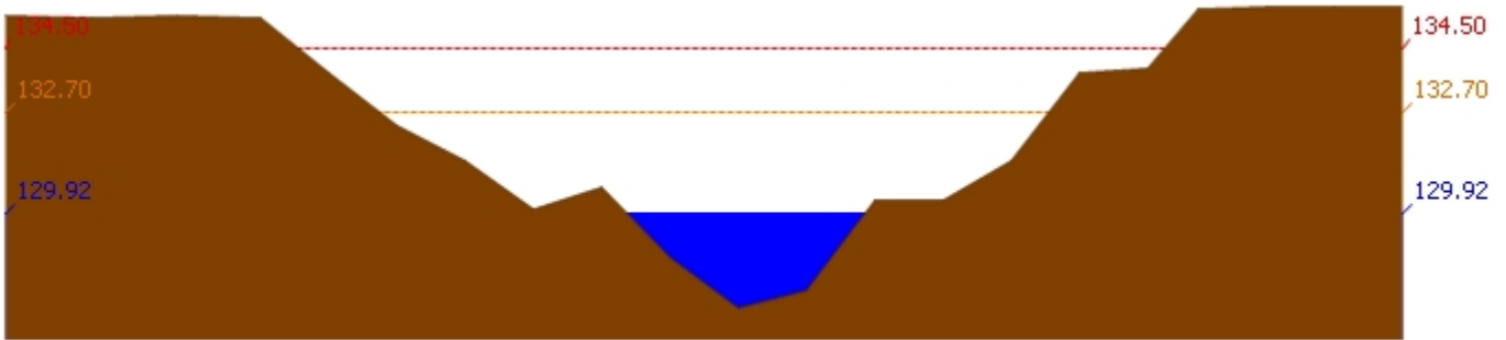
สถานี 120111T แม่น้ำป่าสักที่บ้านจางวาง ต.ลานบัว อ.หล่มสัก จ.เพชรบูรณ์ ระดับน้ำ 129.92 ม.รทก.
