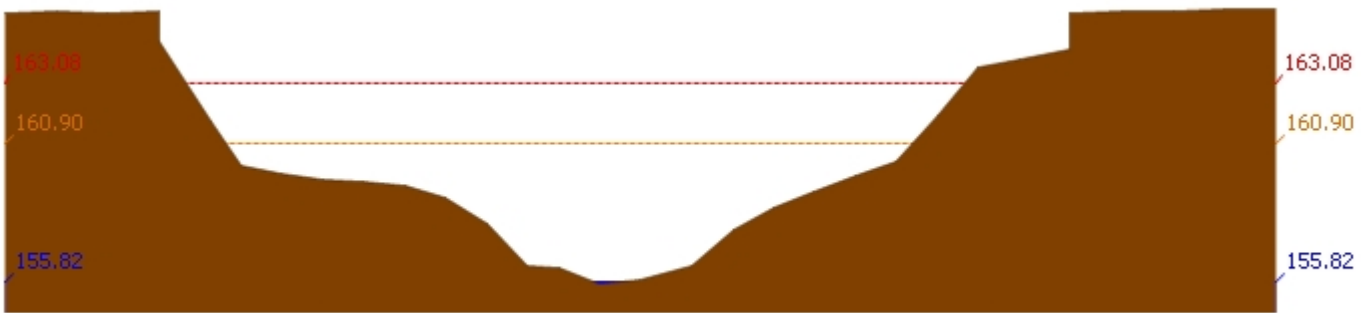
สถานี 120105T แม่น้ำป่าสักที่บ้านวังมเสเหนือ ต.ทำอิบุญ อ.หล่มสัก จ.เพชรบูรณ์ ระดับน้ำ 155.82 ม.รทก.
