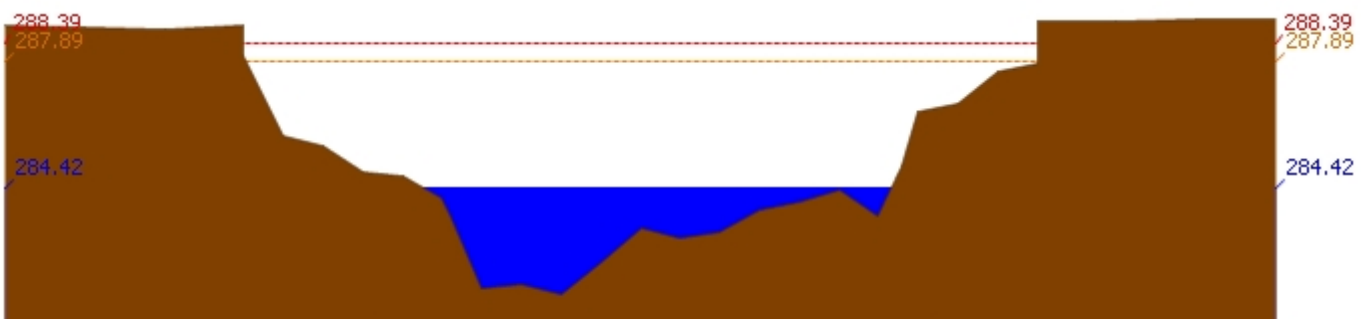
สถานี 070111T แม่น้ำวังที่บ้านโป่งชัย ต.บ้านเสา อ.แจ้ห่ม จ.ลำปาง ระดับน้ำ 284.42 ม.รทก.
