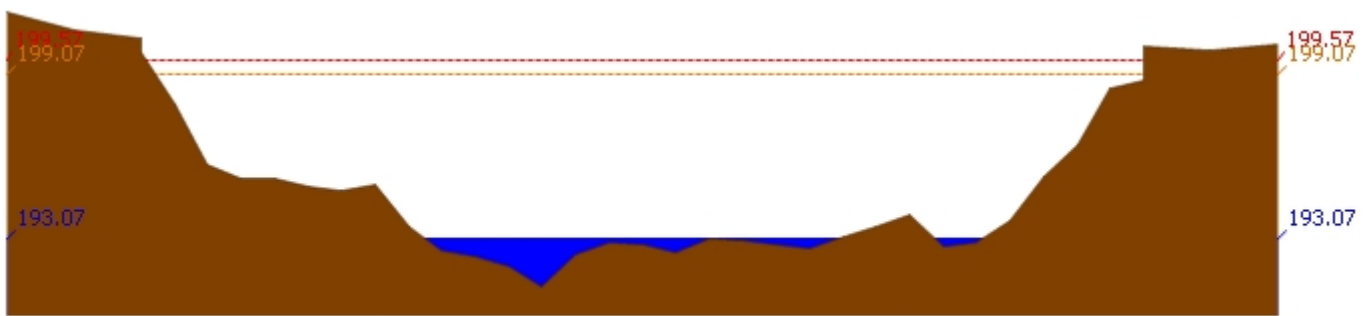
สถานี 070115T น้ำแม่วังที่บ้านอ้อ ต.แม่แก้ว อ.สบปราบ จ.ลำปาง ระดับน้ำ 193.07 ม.รทก.
