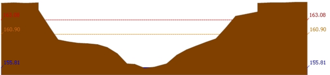
สถานี 120105T แม่น้ำป่าสักที่บ้านวังมเสหนือ ต.ทำอิบุญ อ.หล่มสัก จ.เพชรบูรณ์ ระดับน้ำ 155.81 ม.รทก.
