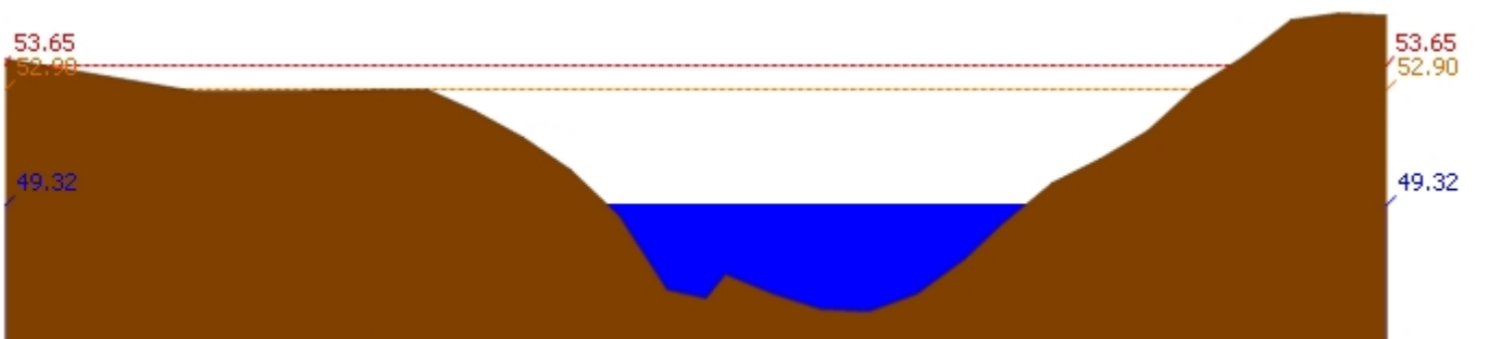
สถานี 120113T แม่น้ำป่าสักที่บ้านเขาค้าง ต.คลองกระจิง อ.ศรีเทพ จ.เพชรบูรณ์ ระดับน้ำ 49.32 ม.รทก.
