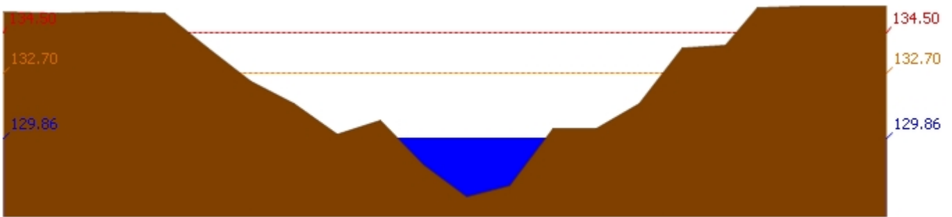
สถานี 120111T แม่น้ำป่าสักที่บ้านจางวาง ต.ลานบัว อ.หล่มสัก จ.เพชรบูรณ์ ระดับน้ำ 129.86 ม.รทก.
