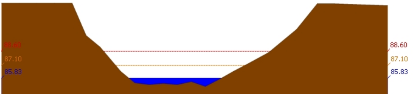
สถานี 120110T แม่น้ำป่าสักที่บ้านวังโบสถ์ ต.วังโบสถ์ อ.หนองไผ่ จ.เพชรบูรณ์ ระดับน้ำ 85.83 ม.รทก.
