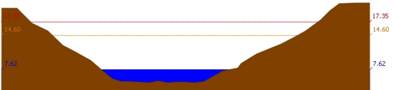
สถานี 120109T แม่น้ำป่าสักที่ อ.แก่งคอย ต.แก่งคอย อ.แก่งคอย จ.สระบุรี ระดับน้ำ 7.62 ม.รทก.
