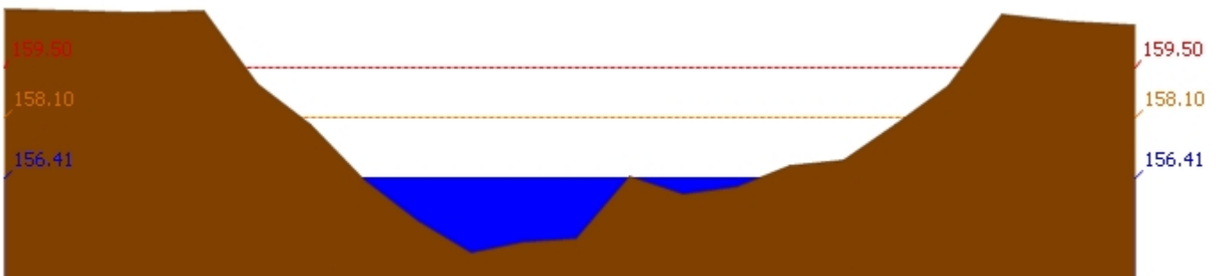
สถานี 120305T หัวน้ำพุที่ อ.หล่มเก่า ต.หล่มเก่า อ.หล่มเก่า จ.เพชรบูรณ์ ระดับน้ำ 156.41 ม.รทก.
