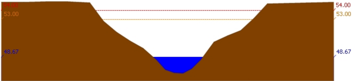
สถานี 120702T ลำสนธิที่บ้านท่าช้าง ต.หนองขาหย่าง อ.ชัยบาดาล จ.ลพบุรี ระดับน้ำ 48.67 ม.รทก.
