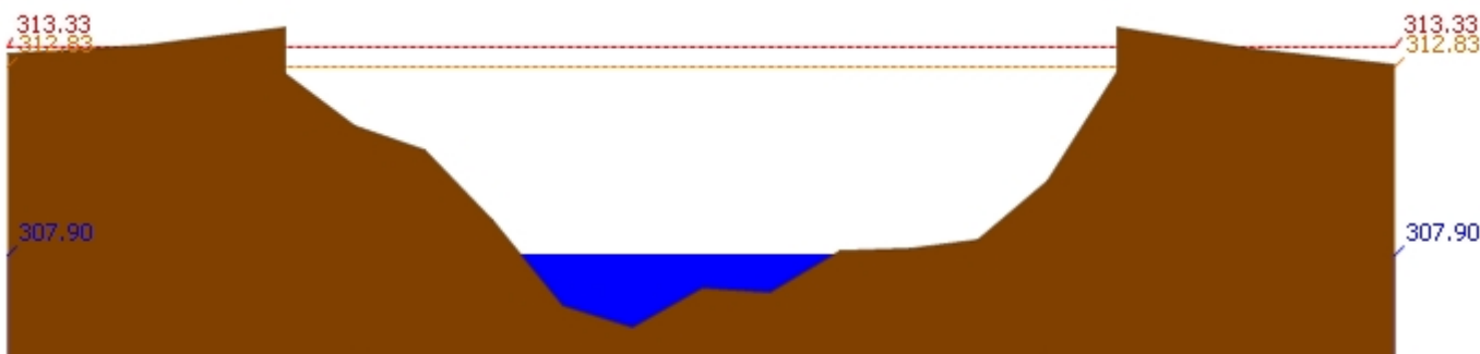
สถานี 060814T น้ำแม่ขานที่บ้านท่าโป่ง ต.บ้านแม อ.สันป่าตอง จ.เชียงใหม่ ระดับน้ำ 307.90 ม.รทก.
