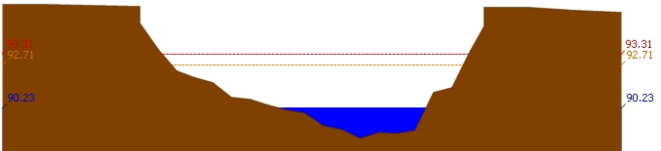
สถานี 061901T คลองแม่ระกาที่บ้านวังชะโอน ต.ท่าไม้ อ.พรานกระต่าย จ.กำแพงเพชร ระดับน้ำ 90.23 ม.รทก.
