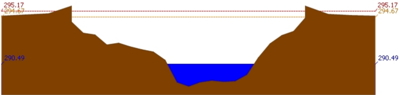
สถานี 060709T น้ำแม่กวังที่ลำพูน ต.เวียงของ อ.เมือง จ.ลำพูน ระดับน้ำ 290.49 ม.รทก.
