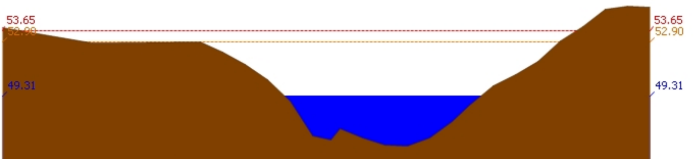
สถานี 120113T แม่น้ำป่าสักที่บ้านเขาค้าง ต.คลองกระจิง อ.ศรีเทพ จ.เพชรบูรณ์ ระดับน้ำ 49.31 ม.รทก.
