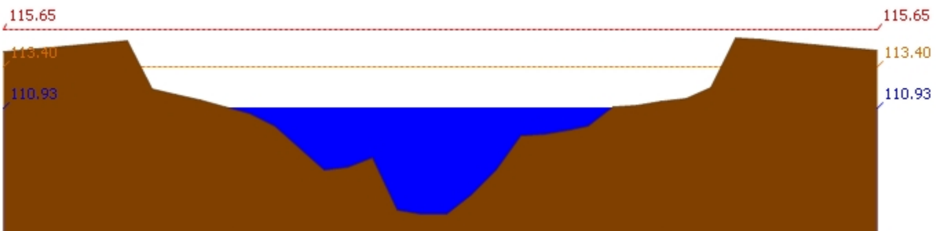
สถานี 120107T แม่น้ำป่าสักที่ อ.เมืองเพชรบูรณ์ ต.นาป่า อ.เมือง จ.เพชรบูรณ์ ระดับน้ำ 110.93 ม.รทก.
