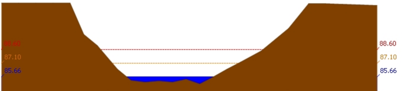
สถานี 120110T แม่น้ำป่าสักที่บ้านวังโบสถ์ ต.วังโบสถ์ อ.หนองไผ่ จ.เพชรบูรณ์ ระดับน้ำ 85.66 ม.รทก.
