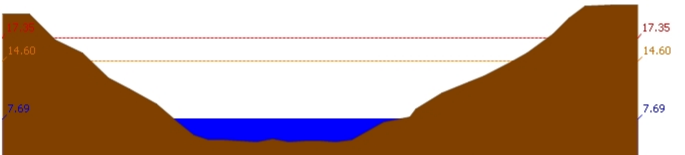
สถานี 120109T แม่น้ำป่าสักที่ อ.แก่งคอย ต.แก่งคอย อ.แก่งคอย จ.สระบุรี ระดับน้ำ 7.69 ม.รทก.
