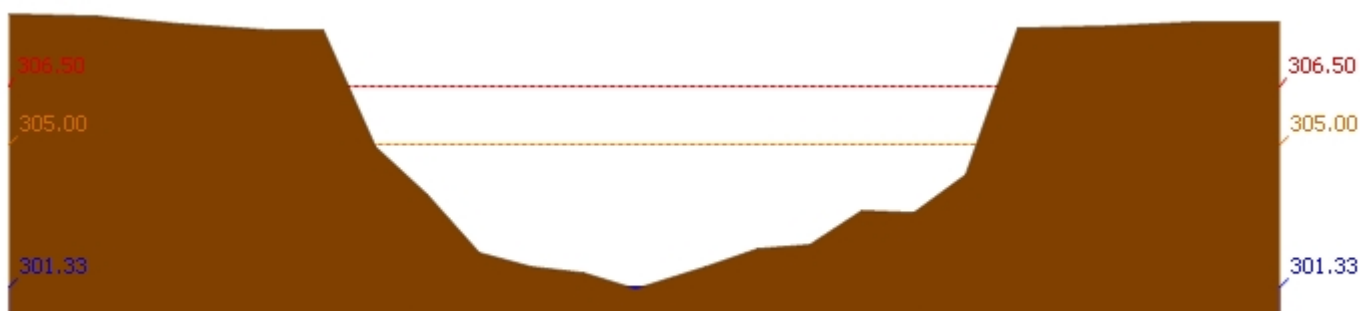
สถานี 120304T ห้วยน้ำพุที่บ้านกกกะบาก ต.โป่ง อ.ด่านซ้าย จ.เลย ระดับน้ำ 301.33 ม.รทก.
