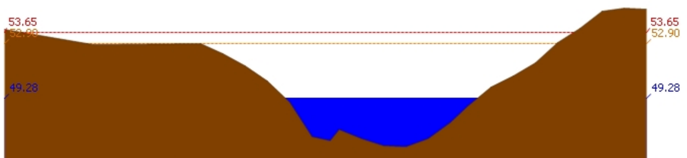
สถานี 120113T แม่น้ำป่าสักที่บ้านเขาค้าง ต.คลองกระจ้ง อ.ศรีเทพ จ.เพชรบูรณ์ ระดับน้ำ 49.28 ม.รทก.
