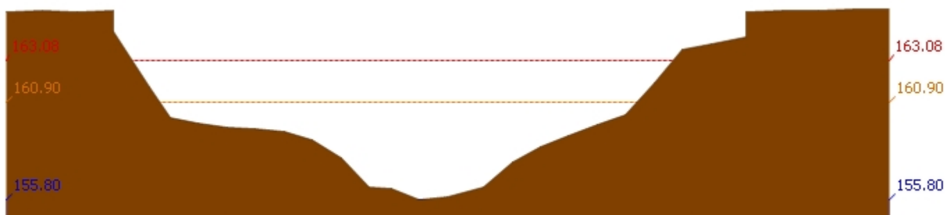
สถานี 120105T แม่น้ำป่าสักที่บ้านวังมสเหนือ ต.ทำอัญญ อ.หล่มสัก จ.เพชรบูรณ์ ระดับน้ำ 155.80 ม.รทก.
