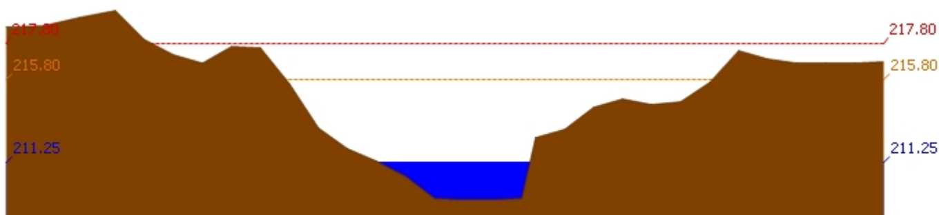
สถานี 120205T แม่น้ำป่าสักที่บ้านอุ้มกะทาด ต.ศิลา อ.หล่มเก่า จ.เพชรบูรณ์ ระดับน้ำ 211.25 ม.รทก.
