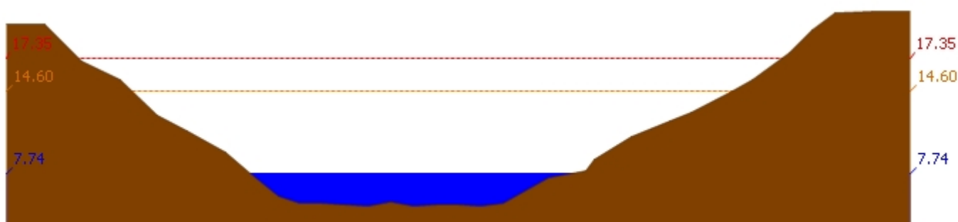
สถานี 120109T แม่น้ำป่าสักที่ อ.แก่งคอย ต.แก่งคอย อ.แก่งคอย จ.สระบุรี ระดับน้ำ 7.74 ม.รทก.
