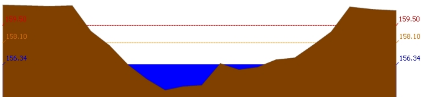
สถานี 120305T หัวขนาฟ่งที่ อ.หล่มเก่า ต.หล่มเก่า อ.หล่มเก่า จ.เพชรบูรณ์ ระดับน้ำ 156.34 ม.รทก.
