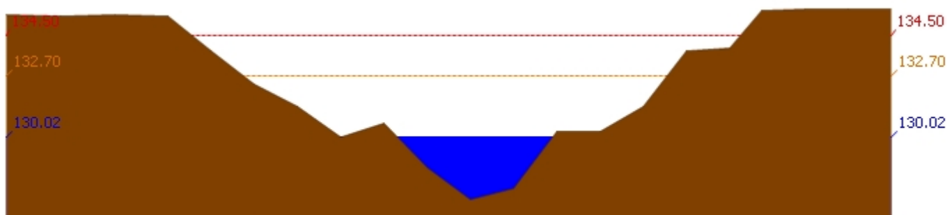
สถานี 120111T แม่น้ำป่าสักที่บ้านจางวาง ต.ลานบัว อ.หล่มสัก จ.เพชรบูรณ์ ระดับน้ำ 130.02 ม.รทก.
