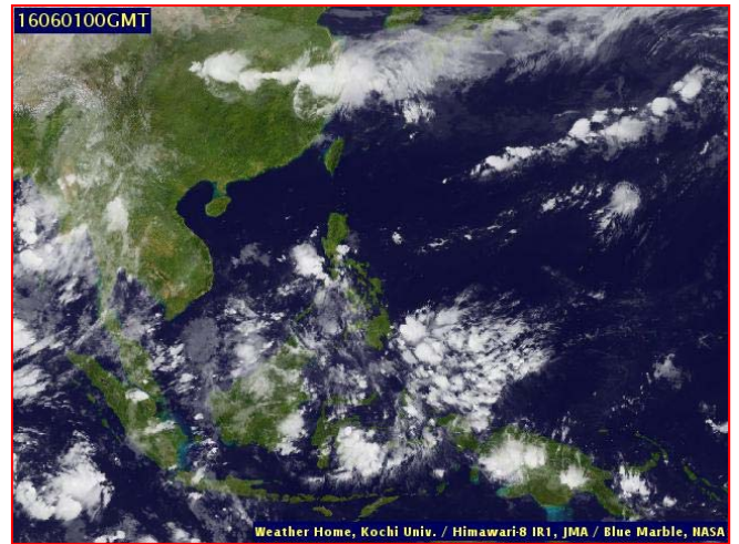
ภาพถ่ายจากดาวเทียม วันที่ ๑ มิ.ย. ๒๕๕๙ เวลา ๐๗.๐๐ น.
