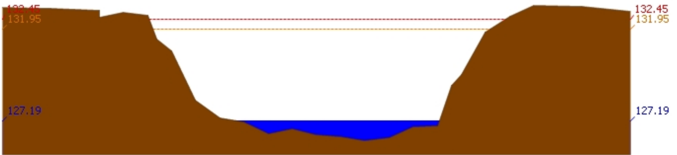
สถานี 070118T แม่น้ำวังที่บ้านแม่สลิด ต.แม่สลิด อ.บ้านตาก จ.ตาก ระดับน้ำ 127.19 ม.รทก.
