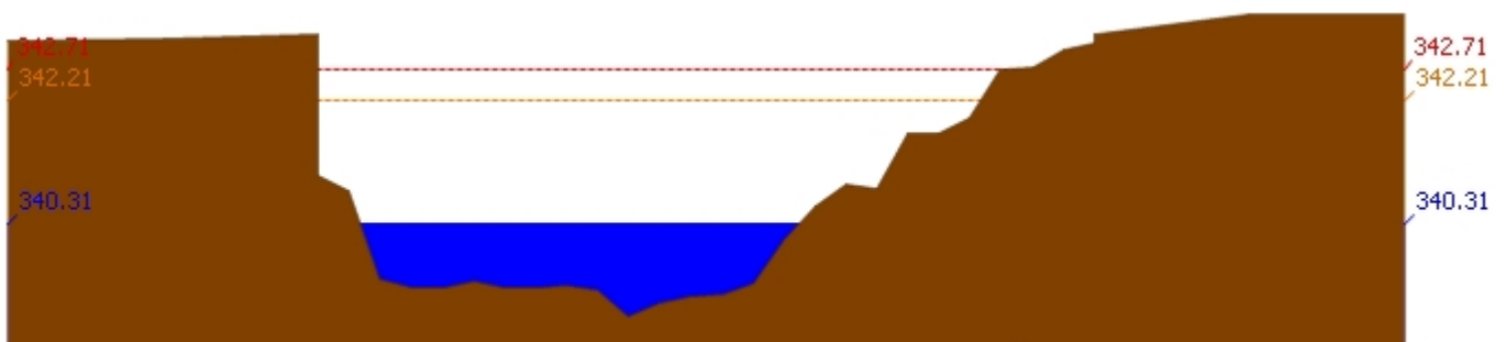
สถานี 070304T น้ำแม่สอยที่บ้านหนองกอก ต.แม่สุก อ.แจ้ห่ม จ.ลำปาง ระดับน้ำ 340.31 ม.รทก.
