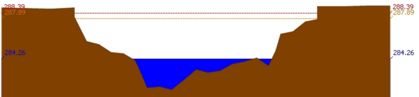
สถานี 070111T แม่น้ำวังที่บ้านโป่งชัย ต.บ้านเสา อ.แจ้ห่ม จ.ลำปาง ระดับน้ำ 284.26 ม.รทก.
