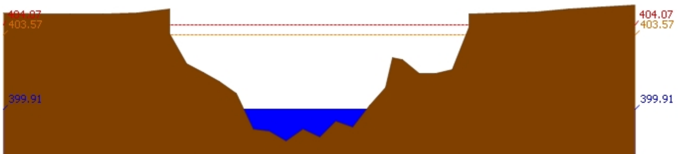
สถานี 070110T แม่น้ำวังที่ อ.วังเหนือ ต.วังเหนือ อ.วังเหนือ จ.ลำปาง ระดับน้ำ 399.91 ม.รทก.
