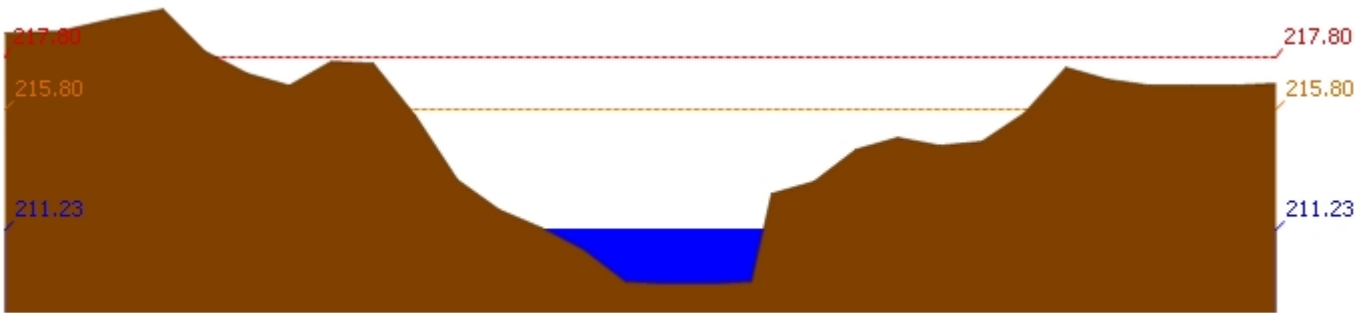
สถานี 120205T แม่น้ำป่าสักที่บ้านอู่กะทาด ต.ศิลา อ.หล่มเก่า จ.เพชรบูรณ์ ระดับน้ำ 211.23 ม.รทก.
