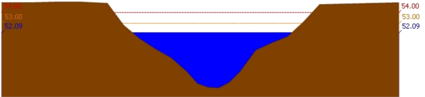
สถานี 120702T ลำสนธิที่บ้านท่าช้าง ต.หนองขาหย่าง อ.ชัยบาดาล จ.ลพบุรี ระดับน้ำ 52.09 ม.รทก.
