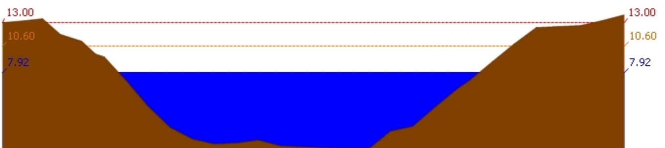
สถานี 120106T แม่น้ำป่าสักที่ อ.เสนาห์ ต.ศาลาวิไทย อ.เสนาห์ จ.สระบุรี ระดับน้ำ 7.92 ม.รทก.
