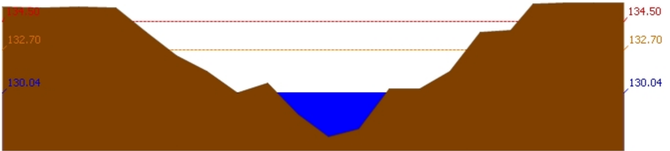
สถานี 120111T แม่น้ำป่าสักที่บ้านจางวาง ต.ลานบัว อ.หล่มสัก จ.เพชรบูรณ์ ระดับน้ำ 130.04 ม.รทก.
