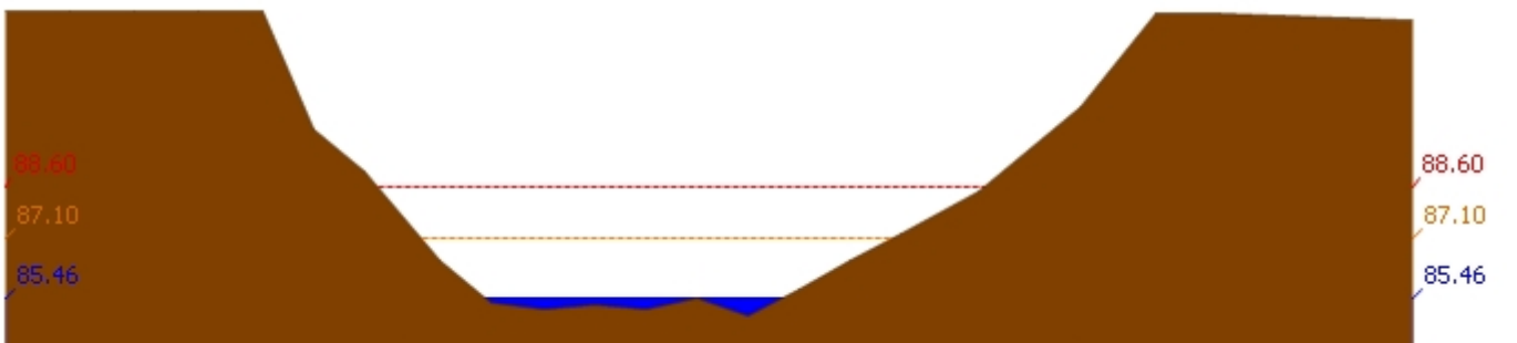
สถานี 120110T แม่น้ำป่าสักที่บ้านวังโบสถ์ ต.วังโบสถ์ อ.หนองไผ่ จ.เพชรบูรณ์ ระดับน้ำ 85.46 ม.รทก.
