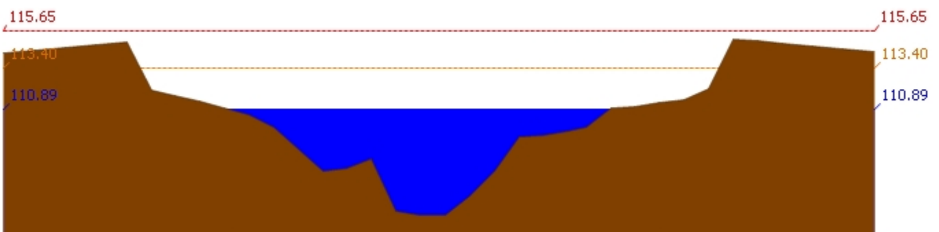
สถานี 120107T แม่น้ำป่าสักที่ อ.เมืองเพชรบูรณ์ ต.นาป่า อ.เมือง จ.เพชรบูรณ์ ระดับน้ำ 110.89 ม.รทก.
