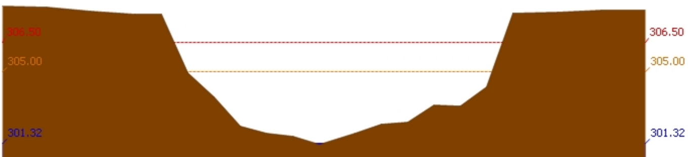
สถานี 120304T ห้วยน้ำพุที่บ้านกกกะบาก ต.โป่ง อ.ด่านซ้าย จ.เลย ระดับน้ำ 301.32 ม.รทก.
