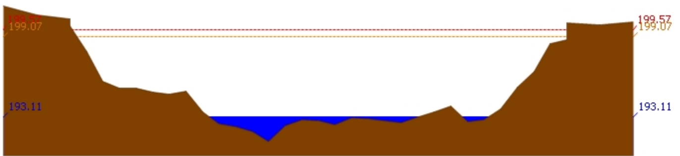
สถานี 070115T น้ำแม่วังที่บ้านอ้อ ต.แม่แก้ว อ.สบปราบ จ.ลำปาง ระดับน้ำ 193.11 ม.รทก.
