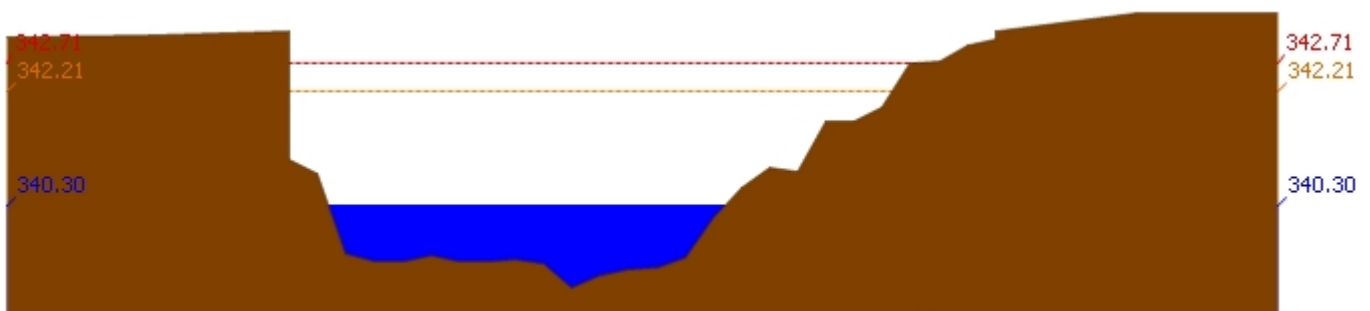
สถานี 070304T น้ำแม่สอยที่บ้านหนองกอก ต.แม่สุก อ.แจ้ห่ม จ.ลำปาง ระดับน้ำ 340.30 ม.รทก.
