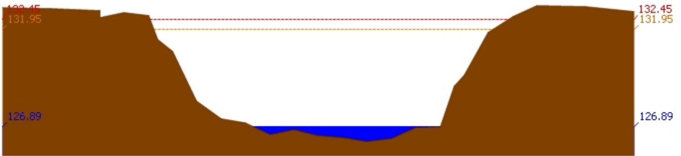
สถานี 070118T แม่น้ำวังที่บ้านแม่สลิด ต.แม่สลิด อ.บ้านตาก จ.ตาก ระดับน้ำ 126.89 ม.รทก.
