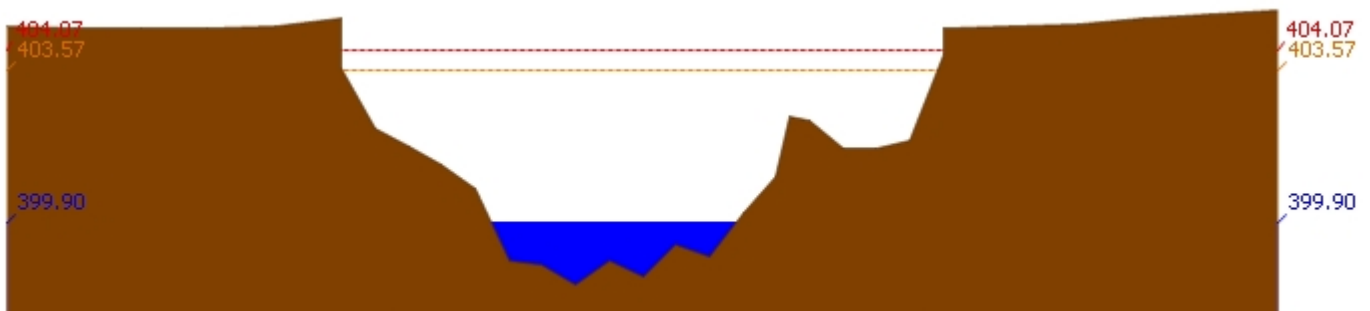
สถานี 070110T แม่น้ำวังที่ อ.วังเหนือ ต.วังเหนือ อ.วังเหนือ จ.ลำปาง ระดับน้ำ 399.90 ม.รทก.
