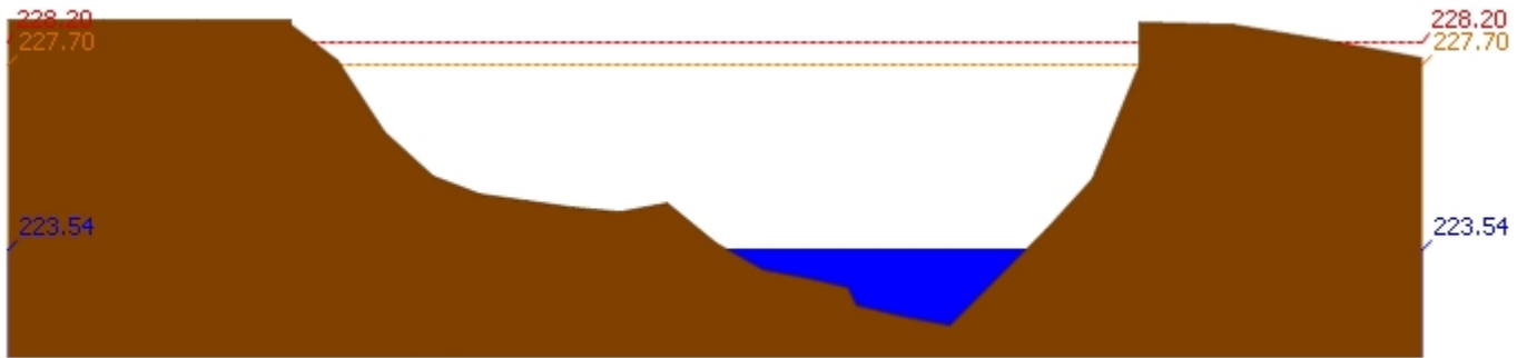
สถานี 070703T น้ำแม่คำที่บ้านนาบอน ต.ทุ่งงาม อ.เสริมงาม จ.ลำปาง ระดับน้ำ 223.54 ม.รทก.
