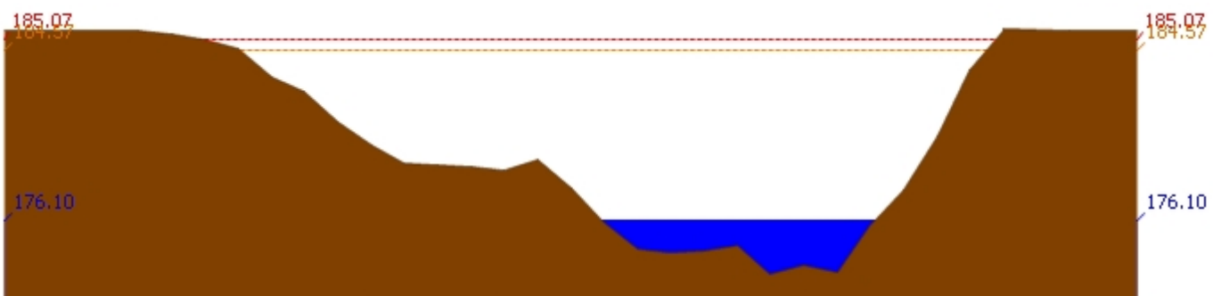
สถานี 070116T แม่น้ำวังที่บ้านแม่เตี๊ยะ ต.แม่ถอด อ.เถิน จ.ลำปาง ระดับน้ำ 176.10 ม.รทก.
