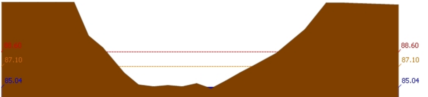
สถานี 120110T แม่น้ำป่าสักที่บ้านวังโบสถ์ ต.วังโบสถ์ อ.หนองไผ่ จ.เพชรบูรณ์ ระดับน้ำ 85.04 ม.รทก.
