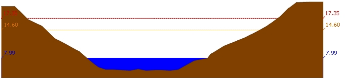
สถานี 120109T แม่น้ำป่าสักที่ อ.แก่งคอย ต.แก่งคอย อ.แก่งคอย จ.สระบุรี ระดับน้ำ 7.99 ม.รทก.
