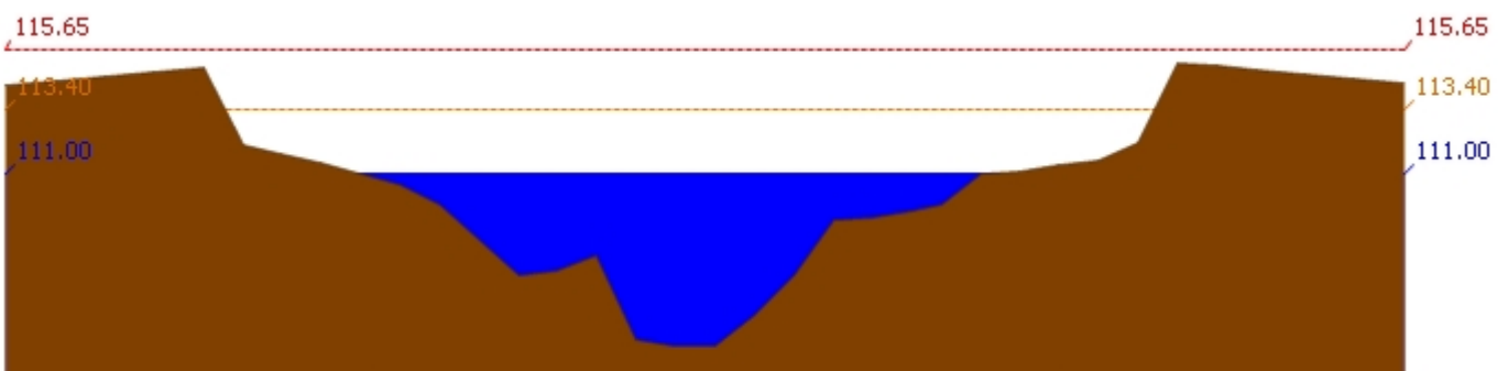
สถานี 120107T แม่น้ำป่าสักที่ อ.เมืองเพชรบูรณ์ ต.นาป่า อ.เมือง จ.เพชรบูรณ์ ระดับน้ำ 111.00 ม.รทก.
