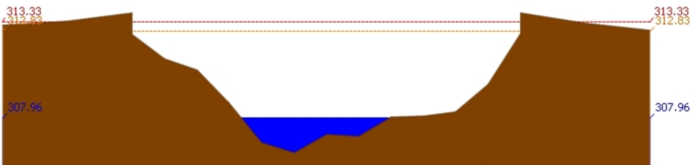
สถานี 060814T น้ำแม่ขานที่บ้านท่าโป่ง ต.บ้านแม อ.สันป่าตอง จ.เชียงใหม่ ระดับน้ำ 307.96 ม.รทก.
