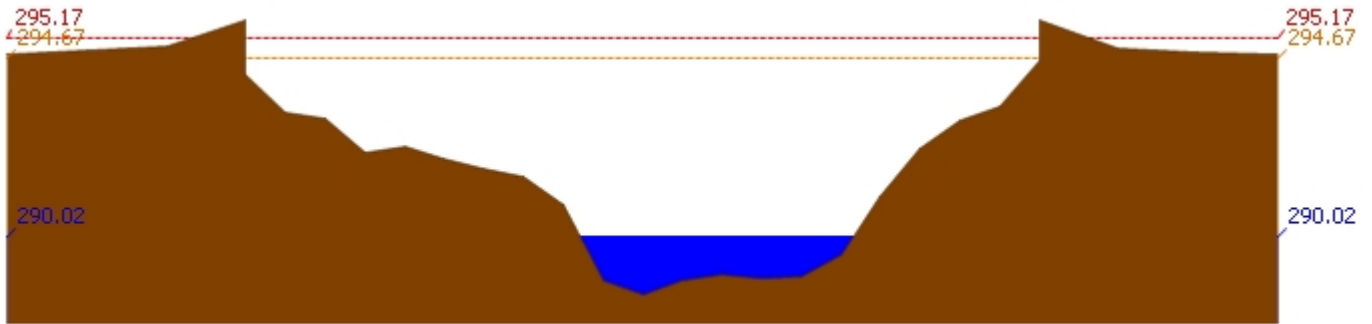
สถานี 060709T น้ำแม่กวังที่ลำพูน ต.เวียงของ อ.เมือง จ.ลำพูน ระดับน้ำ 290.02 ม.รทก.
