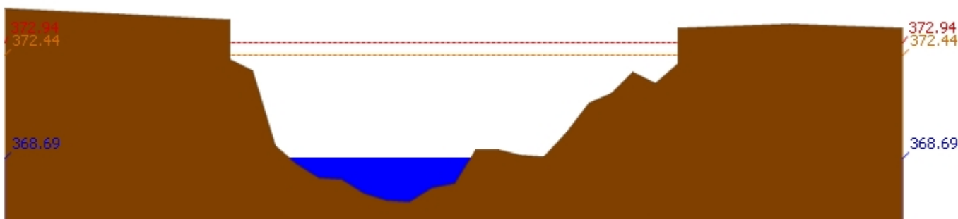
สถานี 060109T แม่น้ำปิงที่บ้านสบอ้อ ต.แม่ระ อ.เชียงดาว จ.เชียงใหม่ ระดับน้ำ 368.69 ม.รทก.
