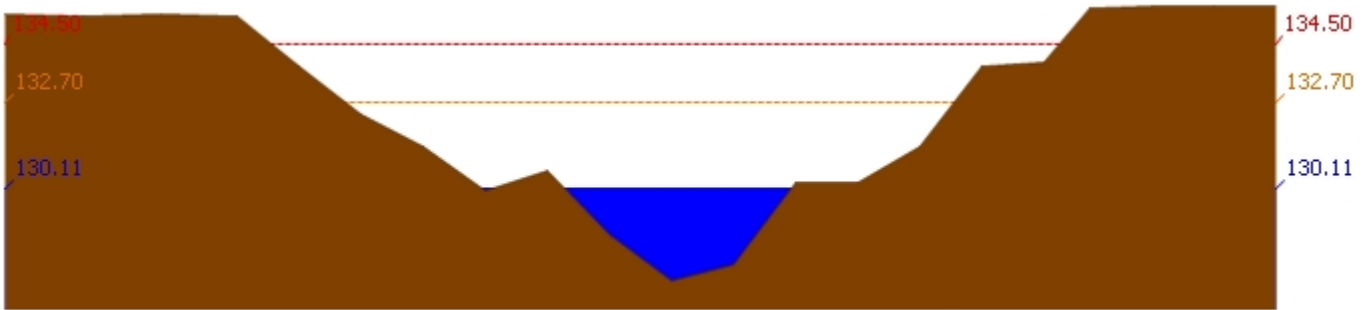
สถานี 120111T แม่น้ำป่าสักที่บ้านจางวาง ต.ลานบัว อ.หล่มสัก จ.เพชรบูรณ์ ระดับน้ำ 130.11 ม.รทก.
