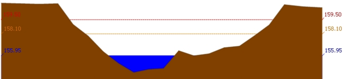
สถานี 120305T หัวน้ำพุที่ อ.หล่มเก่า ต.หล่มเก่า อ.หล่มเก่า จ.เพชรบูรณ์ ระดับน้ำ 155.95 ม.รทก.
