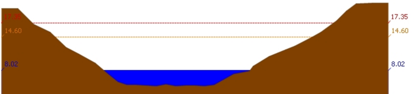
สถานี 120109T แม่น้ำป่าสักที่ อ.แก่งคอย ต.แก่งคอย อ.แก่งคอย จ.สระบุรี ระดับน้ำ 8.02 ม.รทก.
