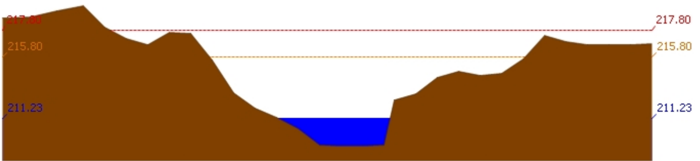
สถานี 120205T แม่น้ำป่าสักที่บ้านอู่กระทาด ต.ศิลา อ.หล่มเก่า จ.เพชรบูรณ์ ระดับน้ำ 211.23 ม.รทก.
