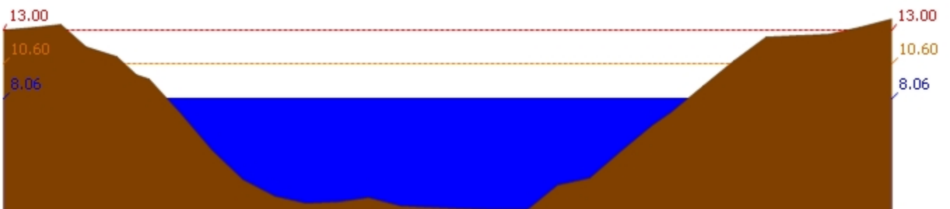
สถานี 120106T แม่น้ำป่าสักที่ อ.เสนาห์ ต.ศาลาวิไทย อ.เสนาห์ จ.สระบุรี ระดับน้ำ 8.06 ม.รทก.
