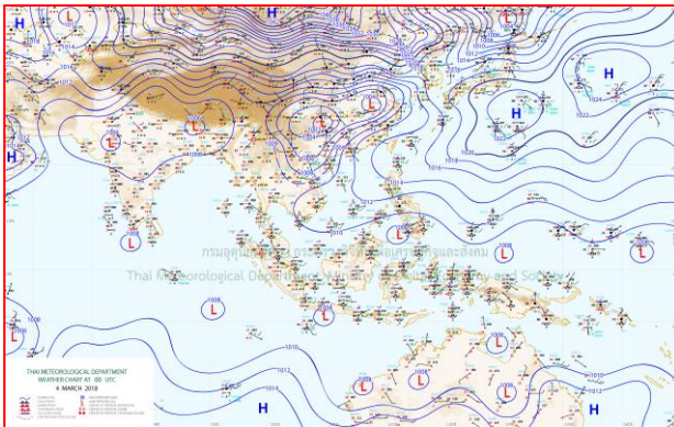
แผนที่อากาศ วันที่ 4 มี.ค. 2561 เวลา 07.00 น.
