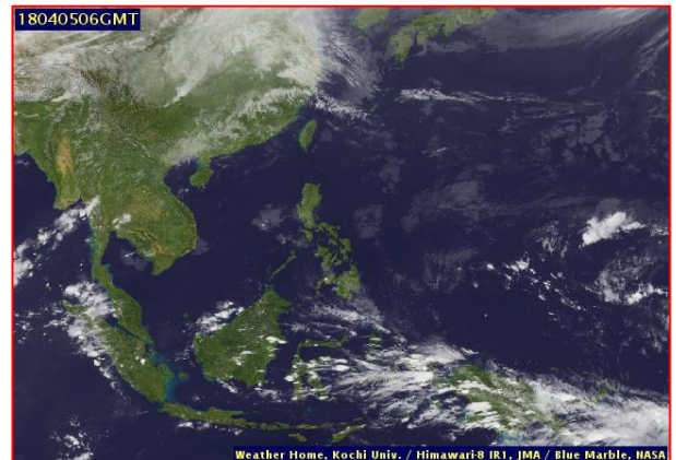
ภาพถ่ายจากดาวเทียม วันที่ ๕ เม.ย. ๒๕๖๑ เวลา ๑๓.๐๐ น.
