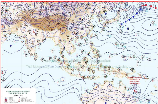
แผนที่อากาศ วันที่ ๕ เม.ย. ๒๕๖๑ เวลา ๐๗.๐๐ น.
