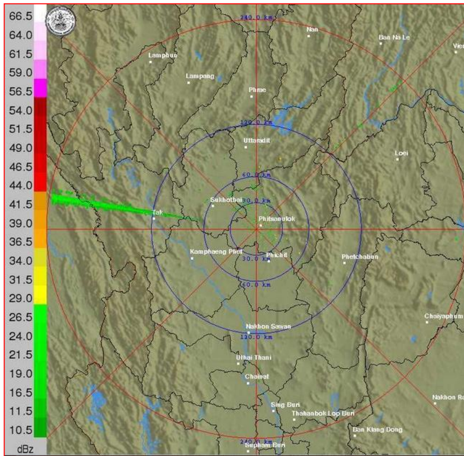
ภาพเรดาร์ตรวจอากาศ “พิชญ์โลก” ณ วันที่ 10 เมษายน 2561 (ที่มา : กรมอุตุนิยมวิทยา)
