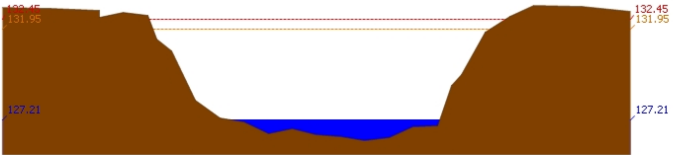
สถานี 070118T แม่น้ำวังที่บ้านแม่สลิด ต.แม่สลิด อ.บ้านตาก จ.ตาก ระดับน้ำ 127.21 ม.รทก.
