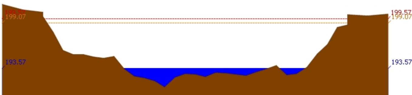
สถานี 070115T น้ำแม่วังที่บ้านอ้อ ต.แม่แก้ว อ.สบปราบ จ.ลำปาง ระดับน้ำ 193.57 ม.รทก.
