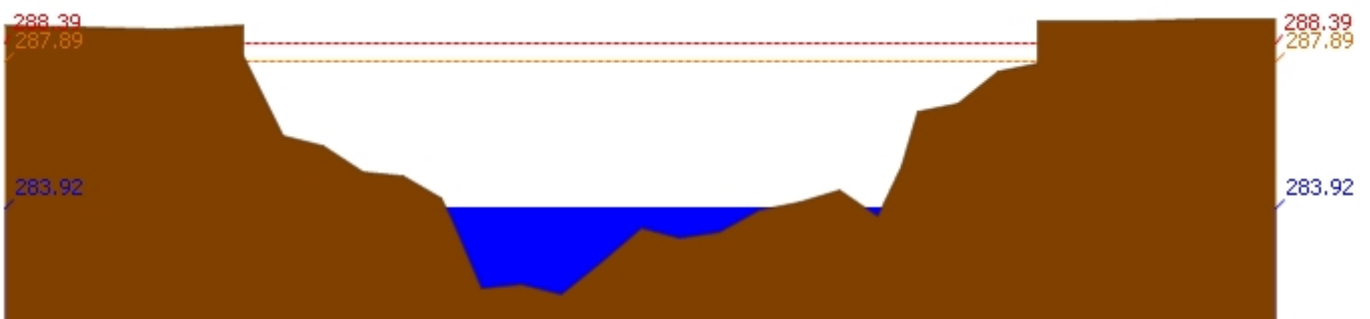
สถานี 070111T แม่น้ำวังที่บ้านเป็นโป่งชัย ต.บ้านเสา อ.แจ้ห่ม จ.ลำปาง ระดับน้ำ 283.92 ม.รทก.
