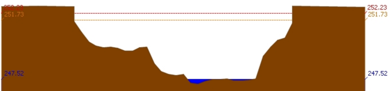
สถานี 070403T น้ำแม่ตุ๋ยที่บ้านแค ต.บ้านเป้า อ.เมืองลำปาง จ.ลำปาง ระดับน้ำ 247.52 ม.รทก.
