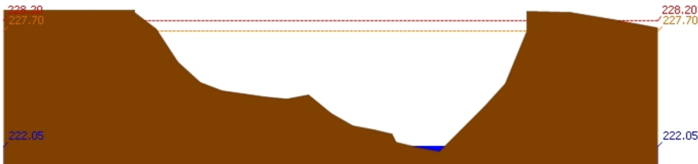
สถานี 070703T น้ำแม่คำที่บ้านนาบอน ต.ทุ่งงาม อ.เสริมงาม จ.ลำปาง ระดับน้ำ 222.05 ม.รทก.
