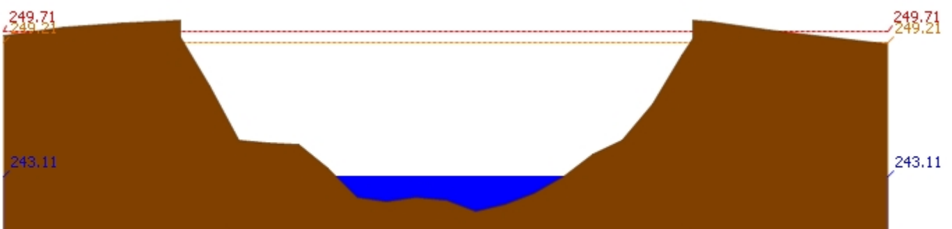
สถานี 070112T แม่น้ำวังที่บ้านบุญนาค ต.บุญนาคพัฒนา อ.เมืองลำปาง จ.ลำปาง ระดับน้ำ 243.11 ม.รทก.
