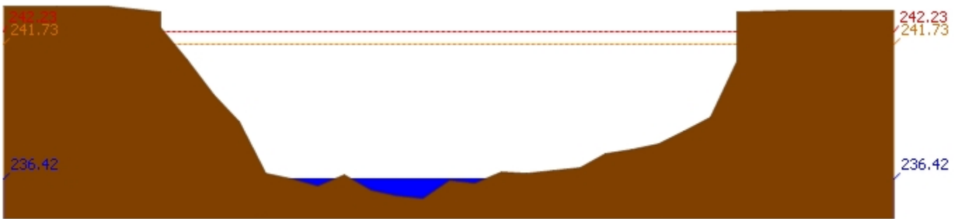
สถานี 070114T แม่น้ำวังที่บ้านปางชัย ต.บ้านเสด็จ อ.เมืองลำปาง จ.ลำปาง ระดับน้ำ 236.42 ม.รทก.
