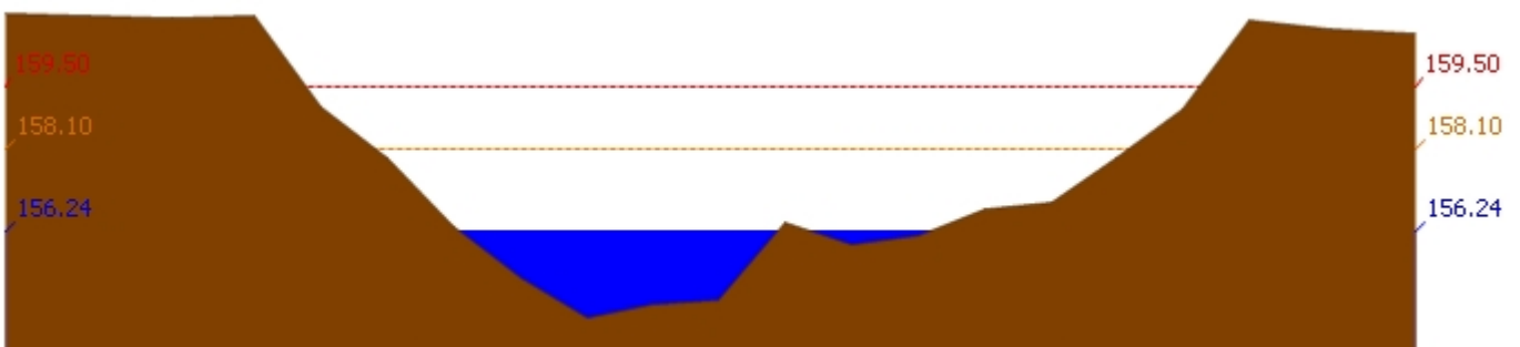
สถานี 120305T หัวน้ำพุที่ อ.หล่มเก่า ต.หล่มเก่า อ.หล่มเก่า จ.เพชรบูรณ์ ระดับน้ำ 156.24 ม.รทก.
