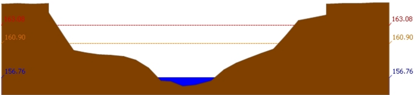
สถานี 120105T แม่น้ำป่าสักที่บ้านวังมเสหนือ ต.ทำอิบุญ อ.หล่มสัก จ.เพชรบูรณ์ ระดับน้ำ 156.76 ม.รทก.
