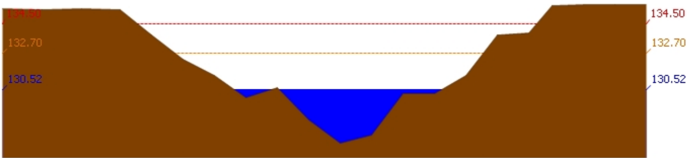
สถานี 120111T แม่น้ำป่าสักที่บ้านจางวาง ต.ลานบัว อ.หล่มสัก จ.เพชรบูรณ์ ระดับน้ำ 130.52 ม.รทก.
