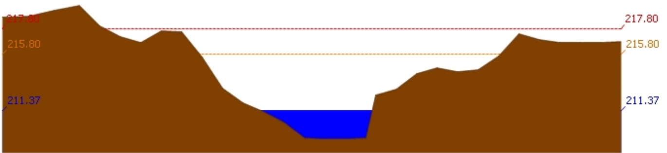
สถานี 120205T แม่น้ำป่าสักที่บ้านอู่กระทาด ต.ศิลา อ.หล่มเก่า จ.เพชรบูรณ์ ระดับน้ำ 211.37 ม.รทก.
