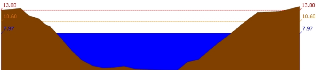
สถานี 120106T แม่น้ำป่าสักที่ อ.เสนาห์ ต.ศาลาวิไทย อ.เสนาห์ จ.สระบุรี ระดับน้ำ 7.97 ม.รทก.
