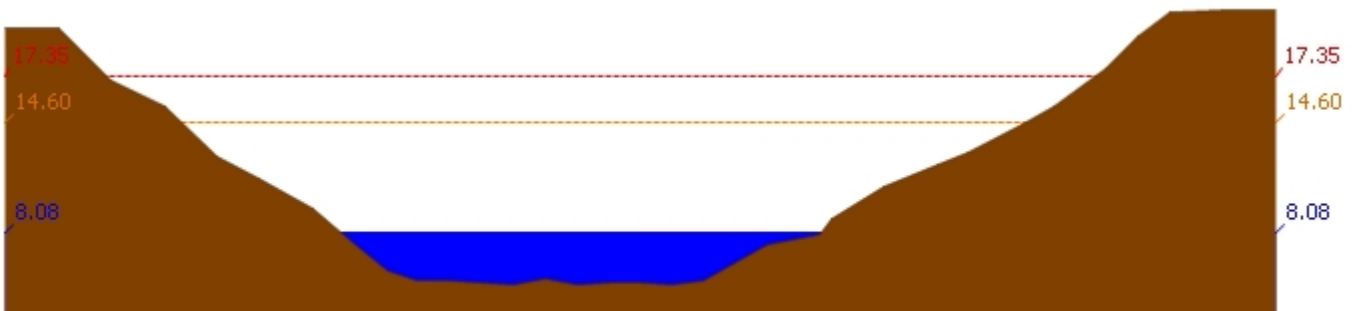
สถานี 120109T แม่น้ำป่าสักที่ อ.แก่งคอย ต.แก่งคอย อ.แก่งคอย จ.สระบุรี ระดับน้ำ 8.08 ม.รทก.
