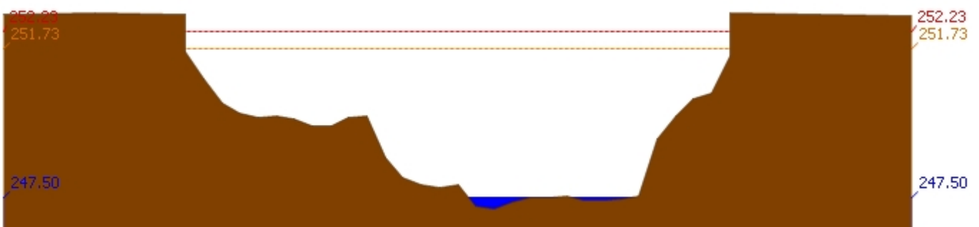
สถานี 070403T น้ำแม่ตุ๋ยที่บ้านแค ต.บ้านเป้า อ.เมืองลำปาง จ.ลำปาง ระดับน้ำ 247.50 ม.รทก.
