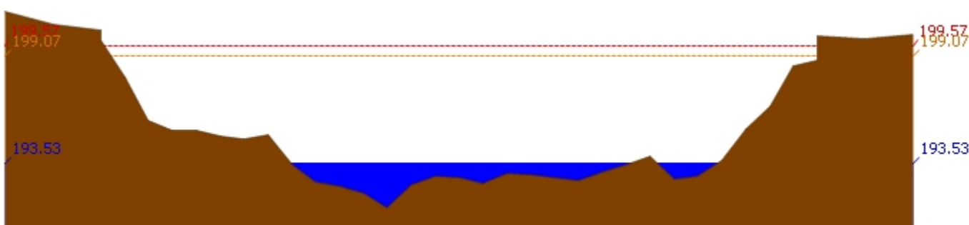
สถานี 070115T น้ำแม่วังที่บ้านอ้อ ต.แม่แก้ว อ.สบปราบ จ.ลำปาง ระดับน้ำ 193.53 ม.รทก.
