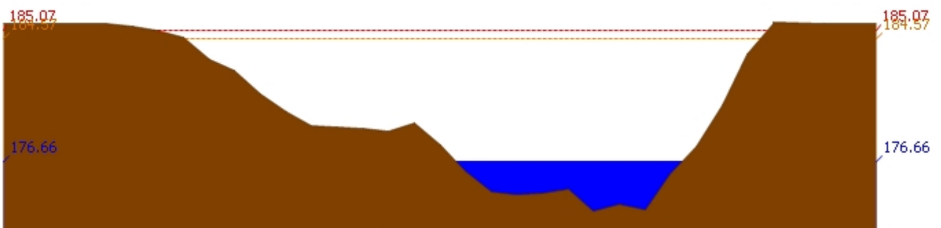
สถานี 070116T แม่น้ำวังที่บ้านแม่เตี๊ยะ ต.แม่ถอด อ.เถิน จ.ลำปาง ระดับน้ำ 176.66 ม.รทก.
