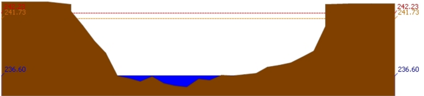
สถานี 070114T แม่น้ำวังที่บ้านปางชัย ต.บ้านเสด็จ อ.เมืองลำปาง จ.ลำปาง ระดับน้ำ 236.60 ม.รทก.
