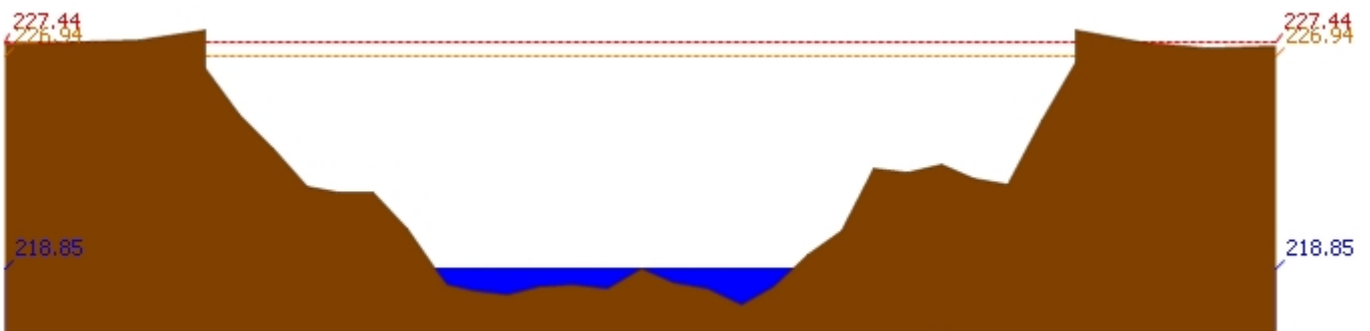
สถานี 070113T แม่น้ำวังที่ จ.ลำปาง ต.เวียงเหนือ อ.เมืองลำปาง จ.ลำปาง ระดับน้ำ 218.85 ม.รทก.
