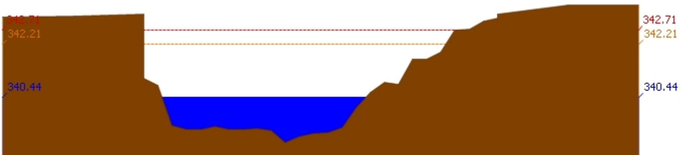
สถานี 070304T น้ำแม่สอยที่บ้านหนองกอก ต.แม่สุก อ.แจ้ห่ม จ.ลำปาง ระดับน้ำ 340.44 ม.รทก.
