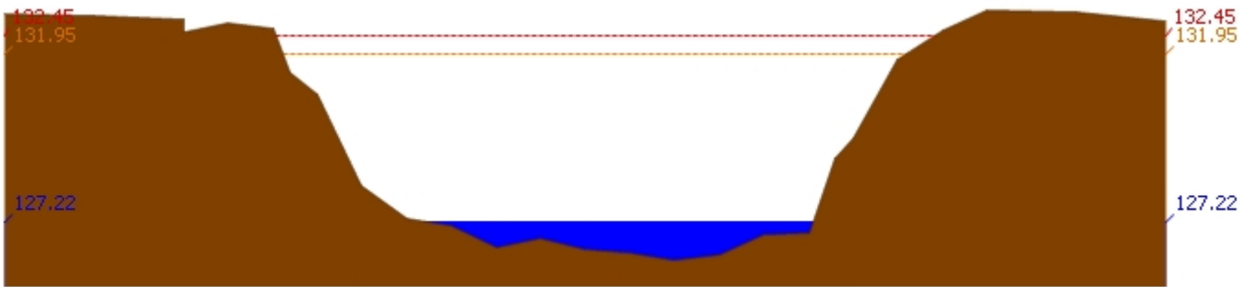
สถานี 070118T แม่น้ำวังที่บ้านแม่สลิด ต.แม่สลิด อ.บ้านตาก จ.ตาก ระดับน้ำ 127.22 ม.รทก.
